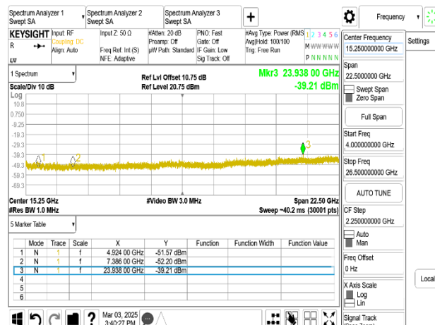
802.11ax_20MHz_Chain0_2462MHz_RU26_8_4-26.5GHz
