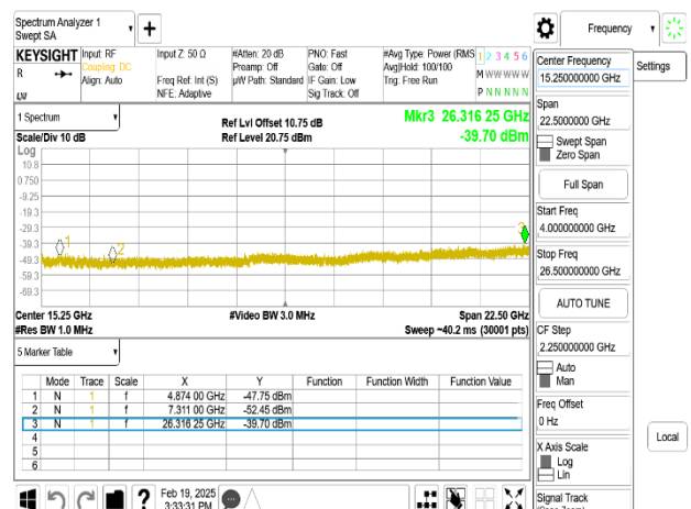
802.11ax_20MHz_Chain0_2437MHz_RU242_4-26.5GHz
