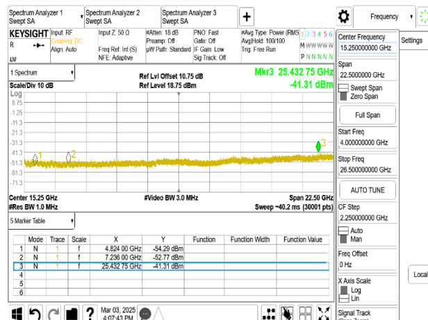
802.11ax_20MHz_Chain0_2412MHz_RU26_0_4-26.5GHz
