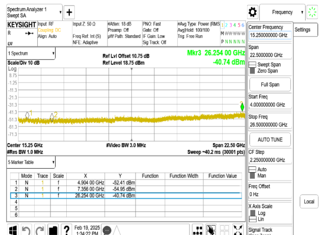
802.11n_40MHz_Chain0_2452MHz_4-26.5GHz
