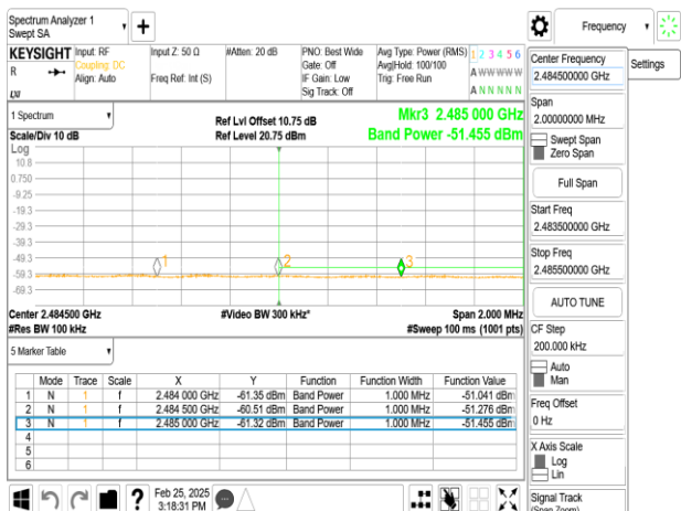
SISO_802.11ax_40MHz_Chain0_2457MHz_RU484
