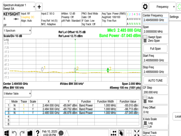
SISO_802.11ax_40MHz_Chain0_2462MHz_RU484
