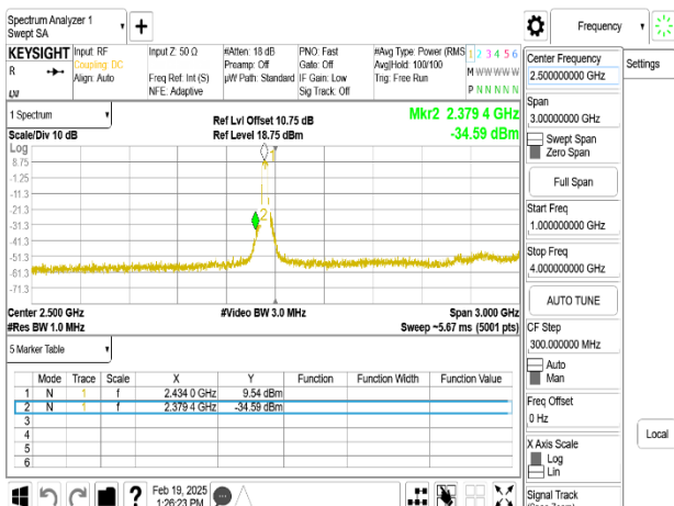
802.11n_40MHz_Chain0_2437MHz_1-4GHz
