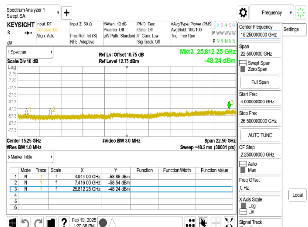
802.11n_20MHz_Chain0_2472MHz_4-26.5GHz
