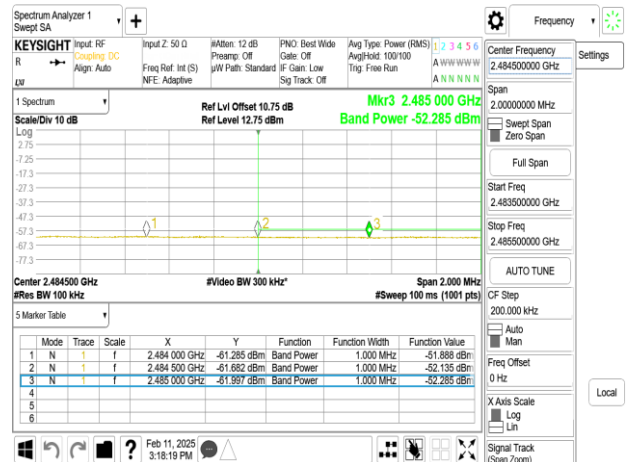
SISO_802.11ax_40MHz_Chain0_2452MHz_RU484
