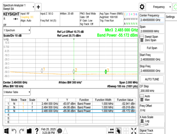
SISO_802.11ax_40MHz_Chain0_2462MHz_RU484
