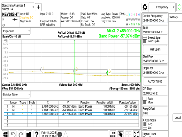
SISO_802.11ax_20MHz_Chain0_2472MHz_RU52_40
