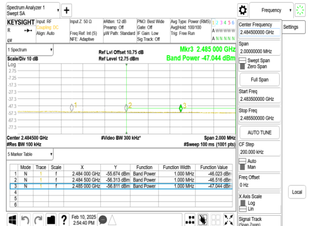
SISO_802.11ax_20MHz_Chain0_2457MHz_RU26_8
