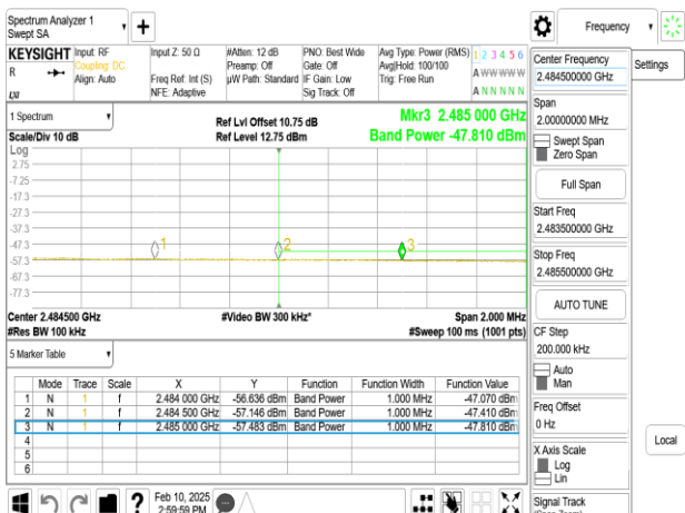
SISO_802.11ax_20MHz_Chain0_2462MHz_RU242
