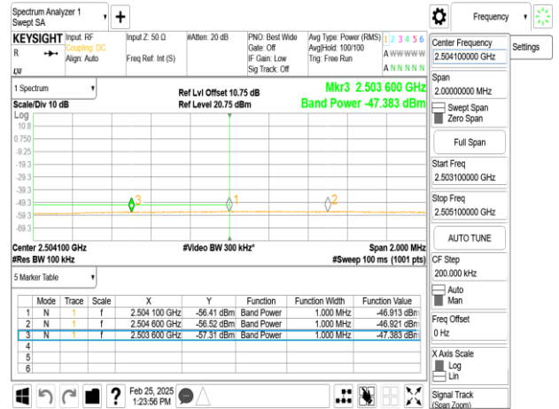
SISO_802.11ax_20MHz_Chain0_2462MHz_RU52_40
