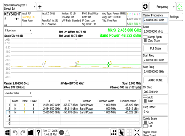
SISO_802.11n_20MHz_Chain0_2462MHz
