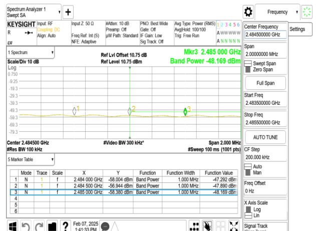
SISO_802.11n_20MHz_Chain0_2462MHz
