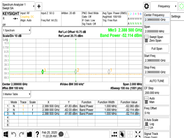
SISO_802.11ax_20MHz_Chain0_2412MHz_RU242
