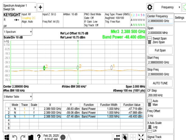
SISO_802.11n_20MHz_Chain0_2417MHz
