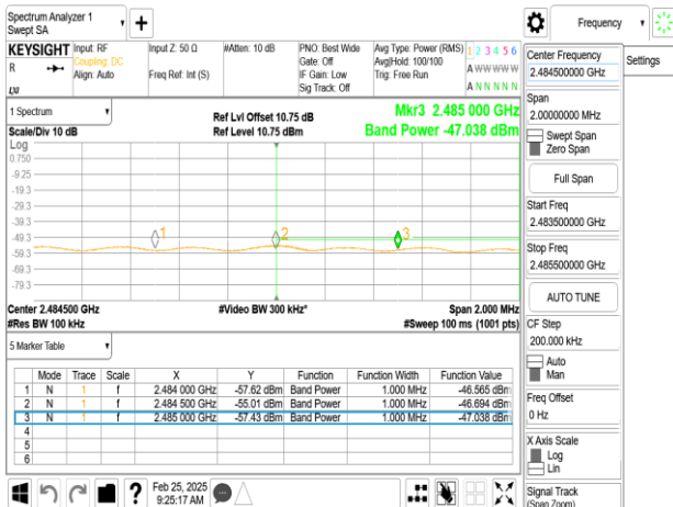
SISO_802.11n_20MHz_Chain0_2472MHz
