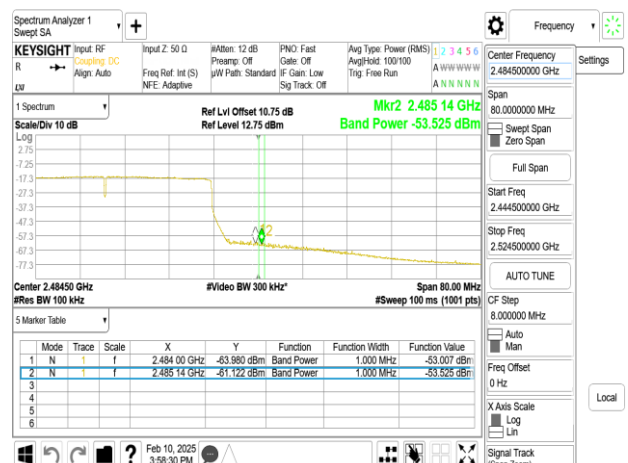
SISO_802.11ax_40MHz_Chain0_2457MHz_RU484
