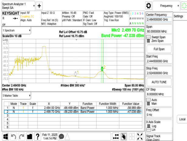
SISO_802.11ax_20MHz_Chain0_2457MHz_RU52_40
