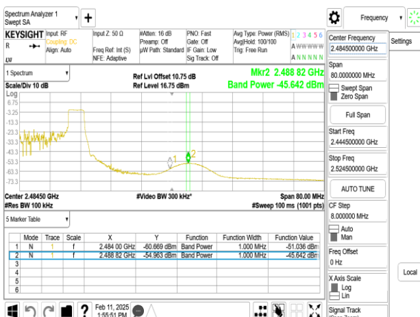
SISO_802.11ax_20MHz_Chain0_2452MHz_RU52_40
