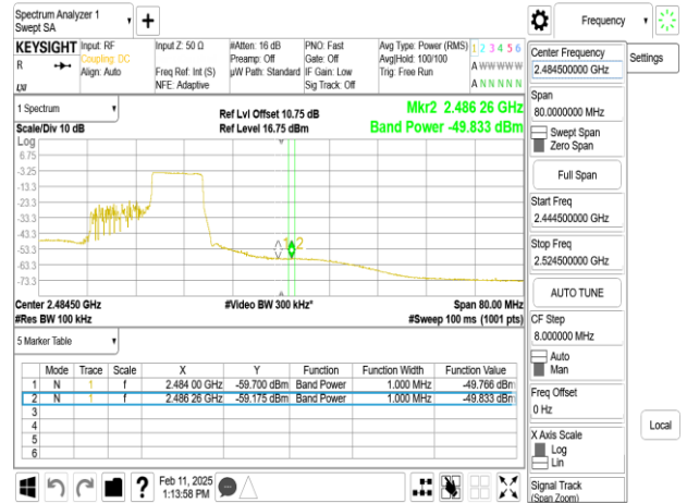
SISO_802.11ax_20MHz_Chain0_2462MHz_RU242
