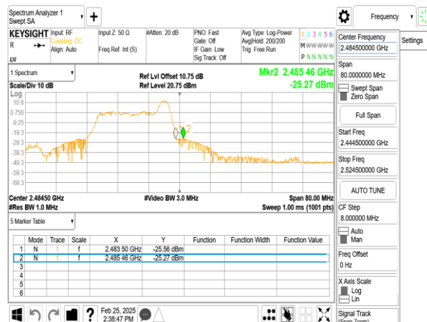
SISO_802.11ax_20MHz_Chain0_2472MHz_RU52_40
