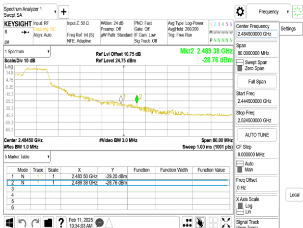
SISO_802.11ax_20MHz_Chain0_2447MHz_RU242
