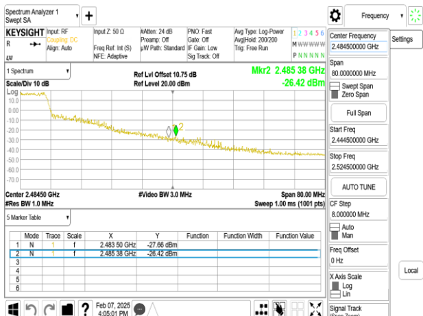
SISO_802.11ax_20MHz_Chain0_2442MHz_RU242
