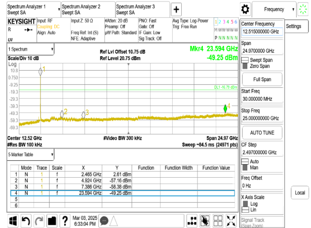
802.11ax_20MHz_Chain0_2462MHz_RU242
