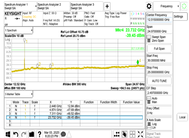
802.11ax_20MHz_Chain0_2437MHz_RU52_40
