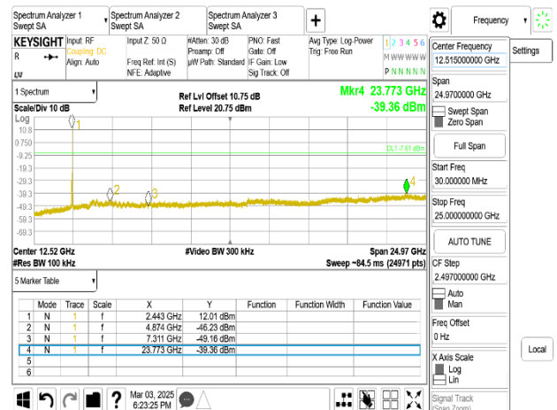
802.11ax_20MHz_Chain0_2437MHz_RU242
