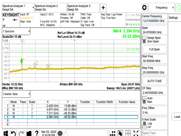
802.11ax_20MHz_Chain0_2437MHz_RU26_0
