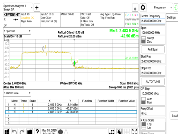
802.11ax_40MHz_Chain0_2462MHz_RU484
