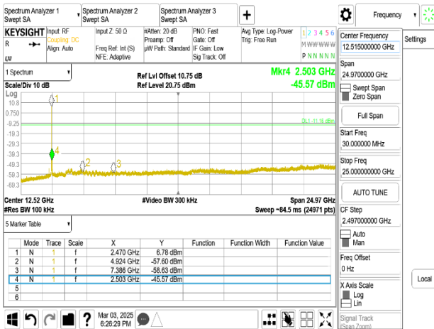
802.11ax_20MHz_Chain0_2462MHz_RU52_40
