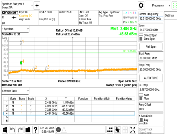
802.11ax_20MHz_Chain0_2462MHz_RU26_8
