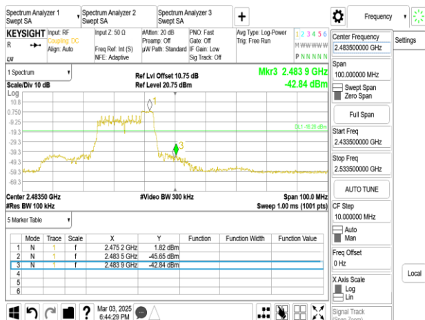
802.11ax_20MHz_Chain0_2472MHz
