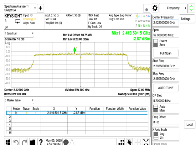
802.11ax_40MHz_Chain0_2422MHz_RU484
