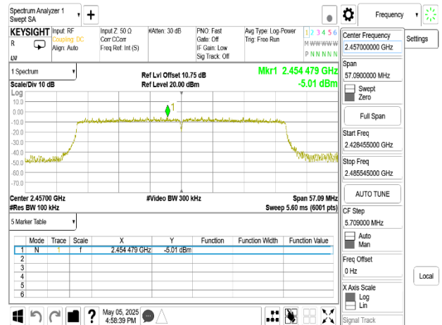
802.11ax_40MHz_Chain0_2457MHz_RU484
