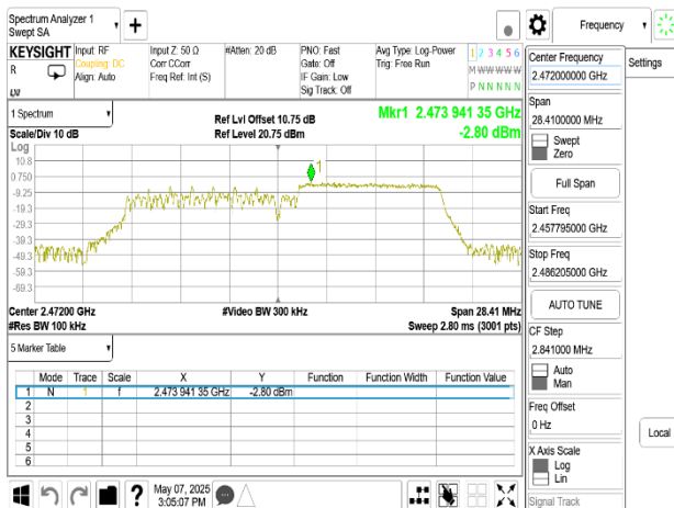
802.11ax_20MHz_Chain0_2472MHz_RU242
