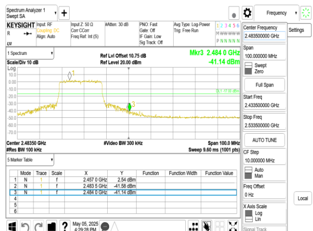
802.11ax_20MHz_Chain0_2462MHz_RU242
