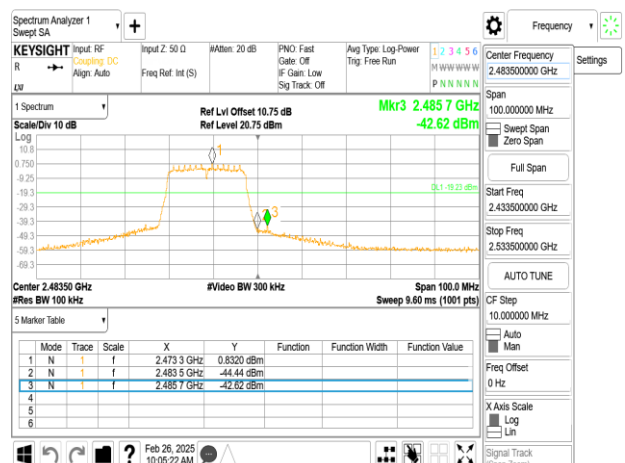
802.11n_20MHz_Chain0_2472MHz
