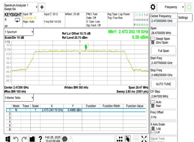
802.11ax_20MHz_Chain0_2472MHz_RU26_8
