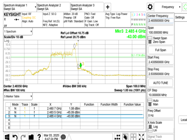
802.11ax_20MHz_Chain0_2472MHz_RU52_40
