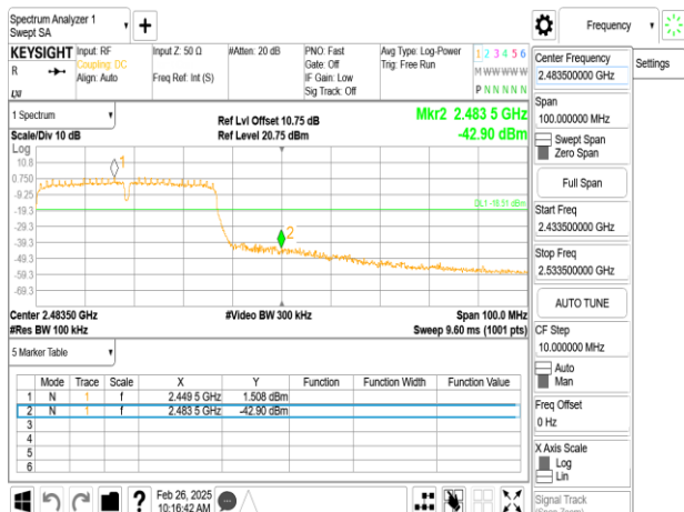
802.11n_40MHz_Chain0_2457MHz
