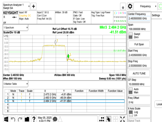
802.11ax_20MHz_Chain0_2472MHz_RU26_8
