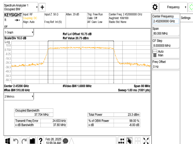
802.11ax_40MHz_Chain0_2452MHz_RU484
