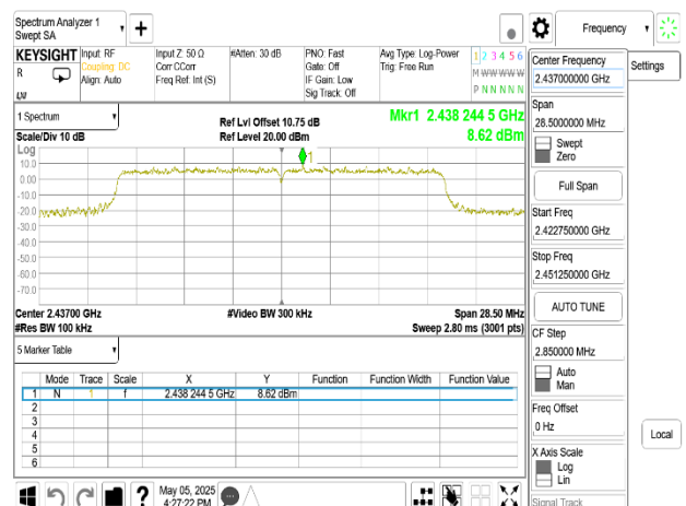
802.11ax_20MHz_Chain0_2437MHz_RU242
