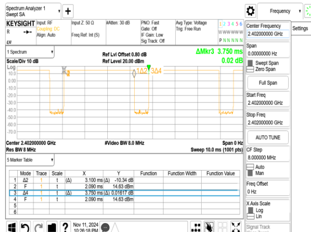
BLE_500k_LowCH00-2402
