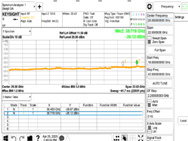
802.11n_20MHz_Chain0_5720MHz_18-40GHz
