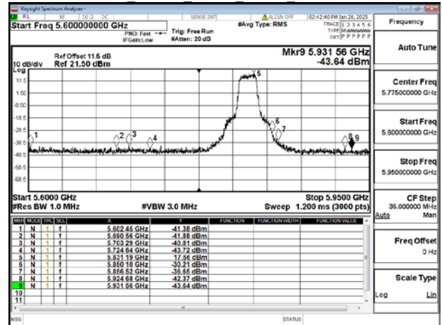
SISO 802.11n 20MHz Chain0 5825MHz
