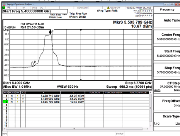
SISO 802.11n 20MHz Chain0 5500MHz
