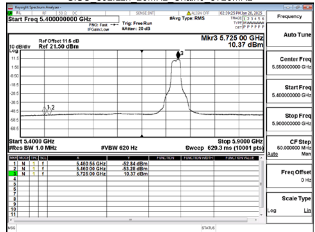
SISO 802.11n 20MHz Chain0 5720MHz
