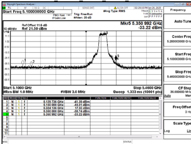
SISO 802.11n 20MHz Chain0 5320MHz
