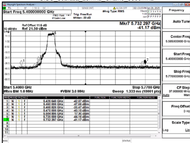
SISO 802.11a 20MHz Chain0 5500MHz
