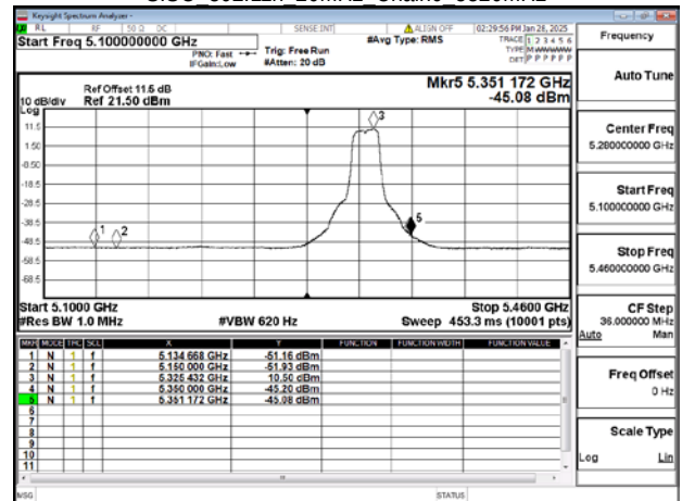
SISO 802.11n 20MHz Chain0 5320MHz
