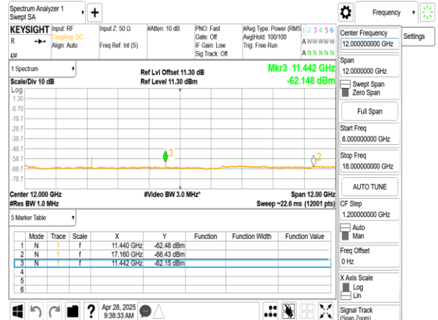
802.11a_20MHz_Chain0_5720MHz_6-18GHz
