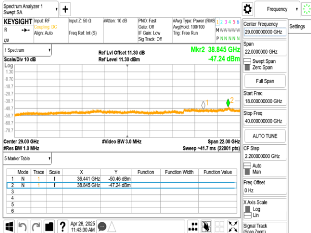
802.11n_20MHz_Chain0_5720MHz_18-40GHz
