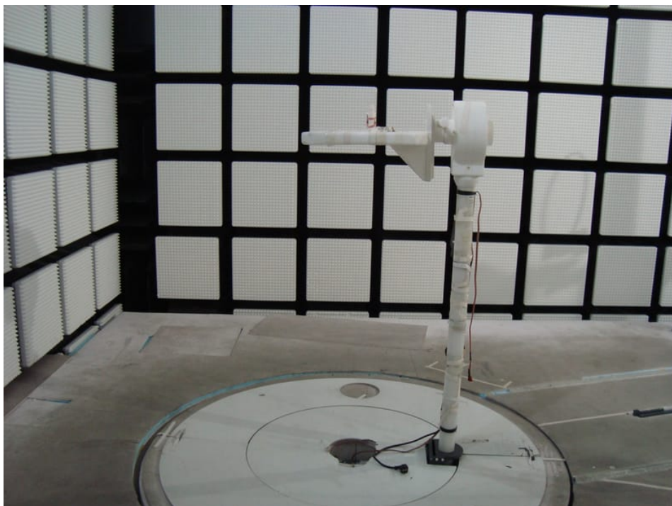
Photo 3: EUT 433 MHz
