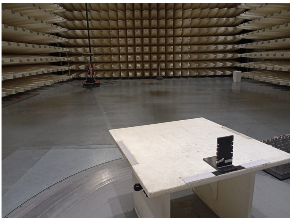
Photo 4: EUT 433 MHz
