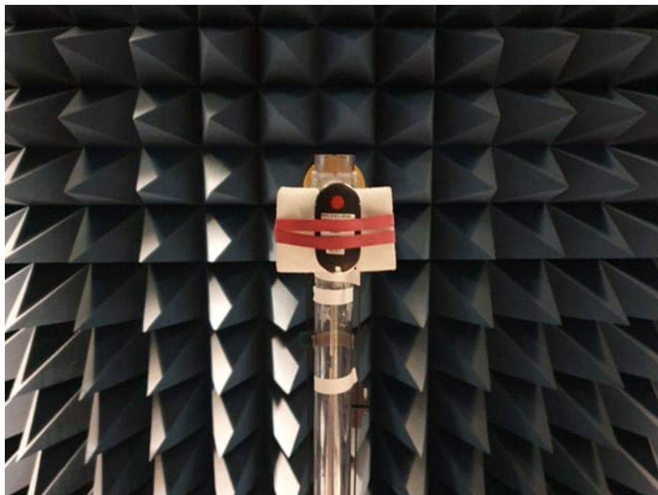
Photo 11: EUT UWB
