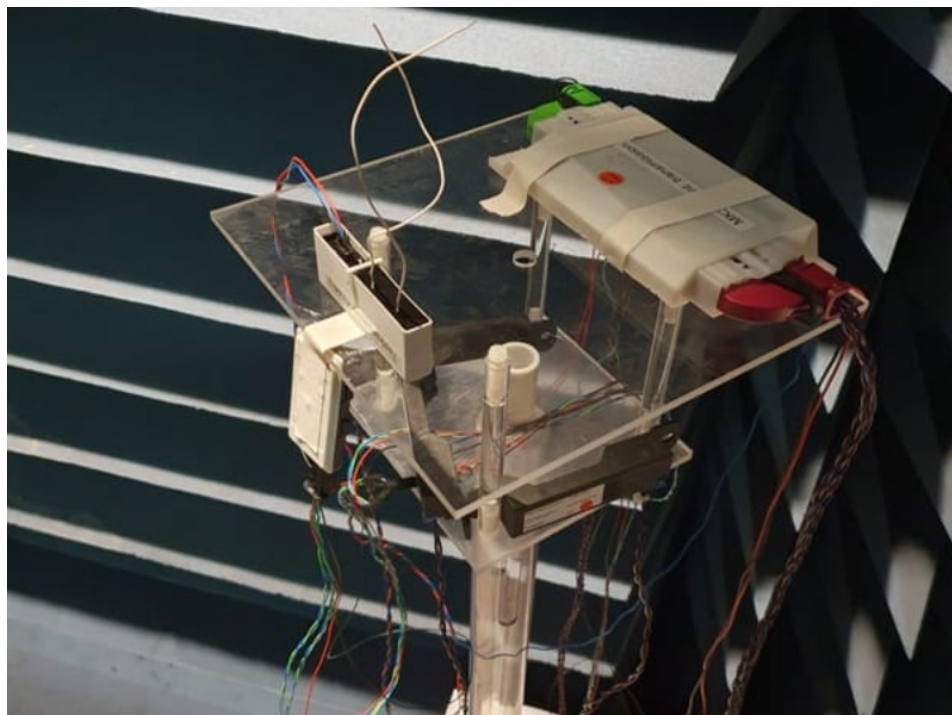
Photo 15: EUT UWB
