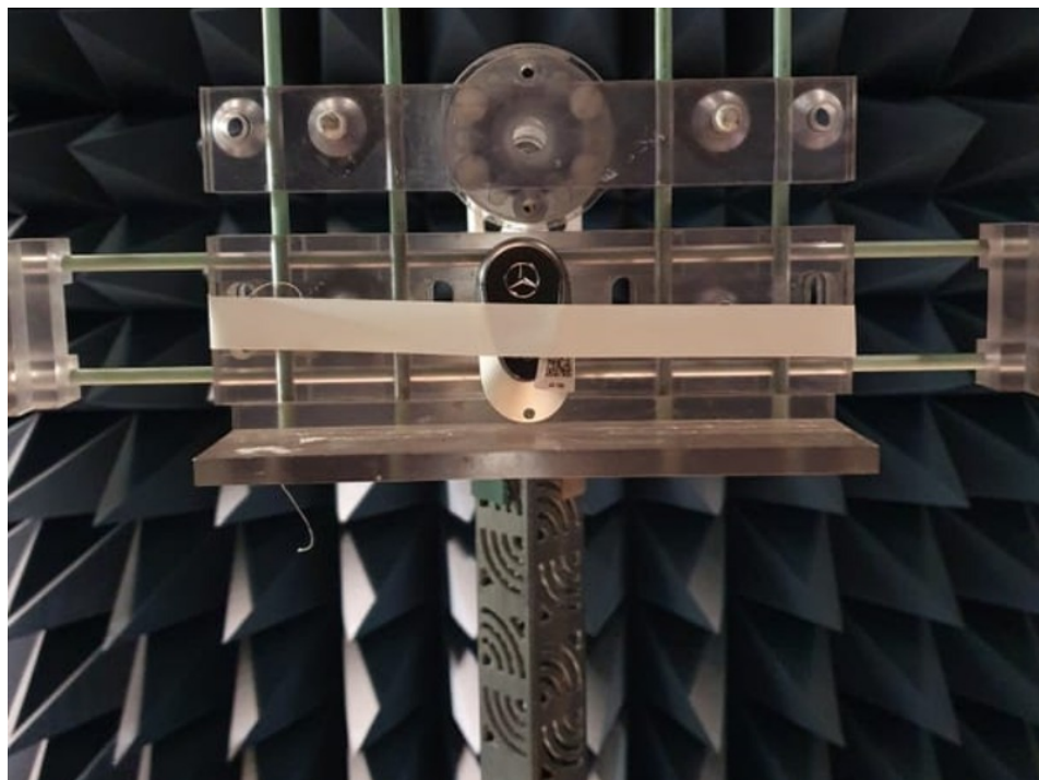
Photo 13: EUT UWB
