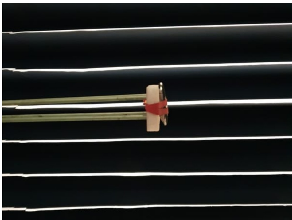
Photo 12: EUT UWB
