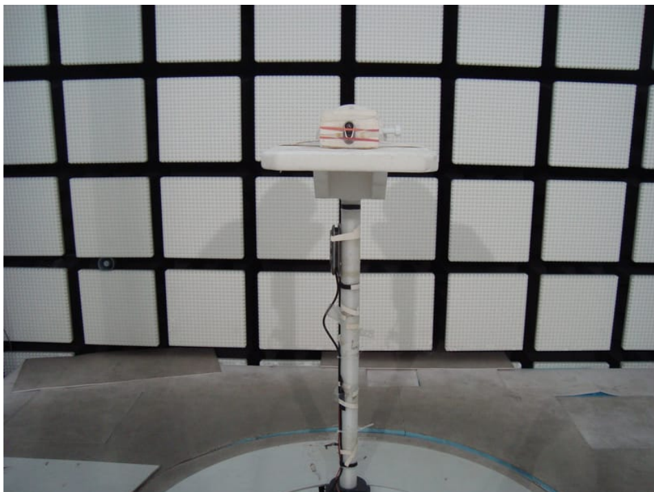
Photo 8: EUT UWB
