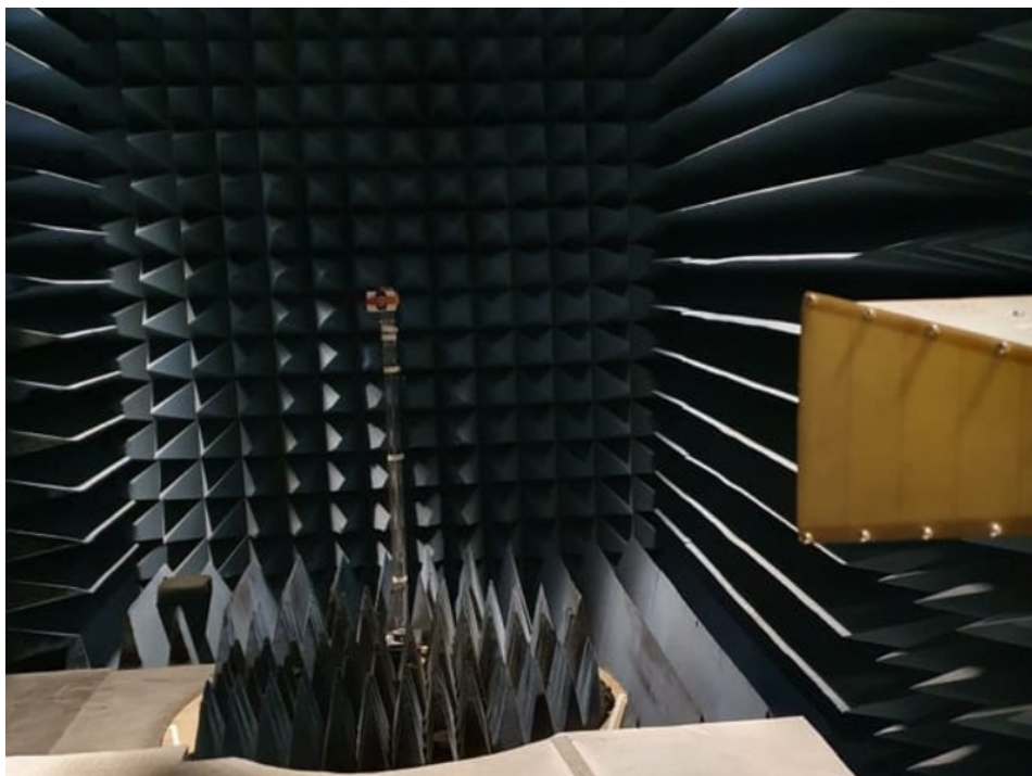
Photo 10: EUT UWB
