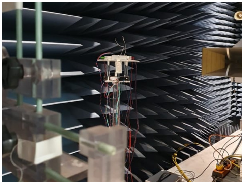
Photo 14: EUT UWB
