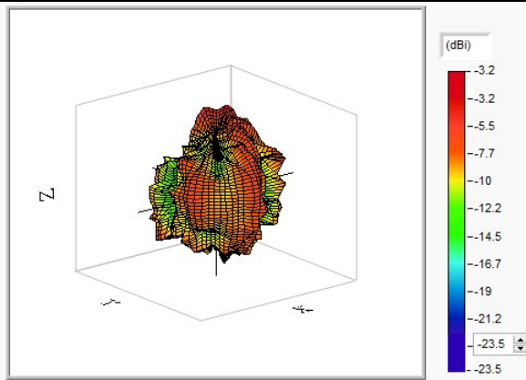
WIFI&BT 5470MHz
