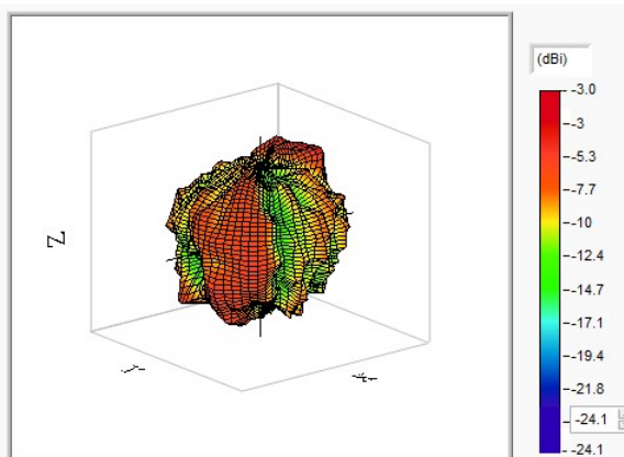
WIFI&BT 5250MHz
