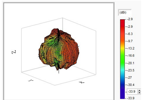
WIFI&BT 5850MHz
