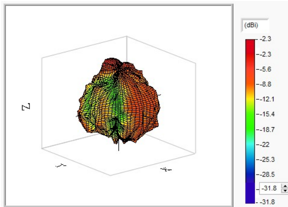
WIFI&BT 5725MHz
