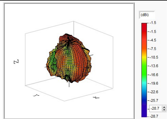
WIFI&BT 5600MHz
