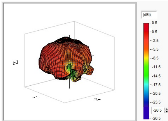
1559MHz
