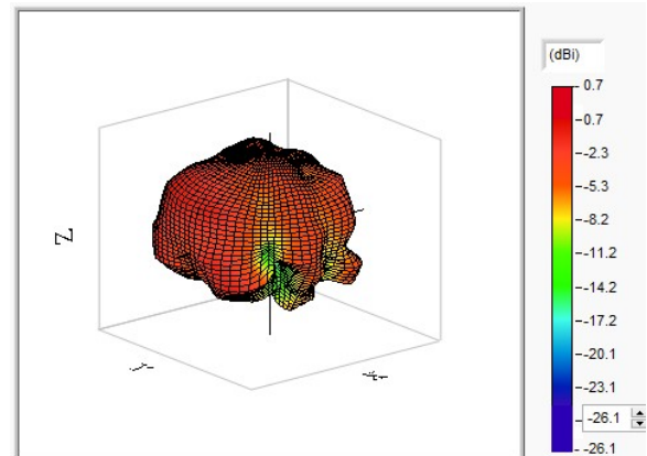
1561MHz
