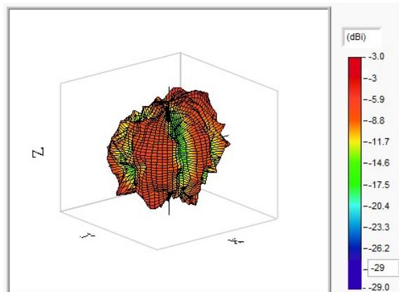
WIFI&BT 5350MHz
