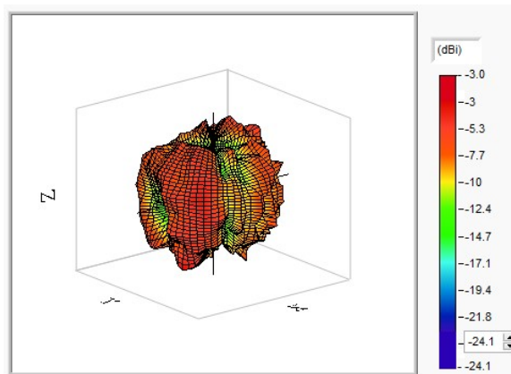
WIFI&BT 5150MHz
