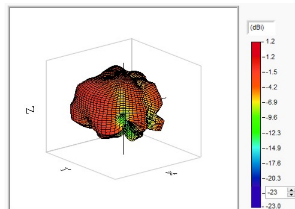
1570MHz
