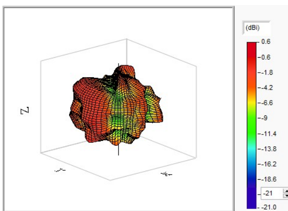
WIFI&BT 2400MHz
