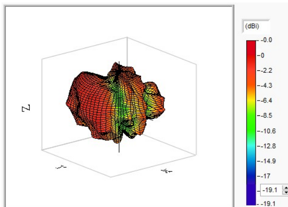
WIFI&BT 2500MHz
