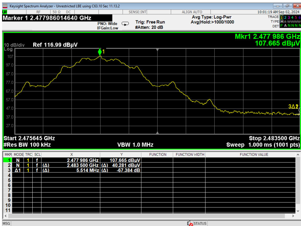
46, HBE Unrestricted, BLE 2MB
