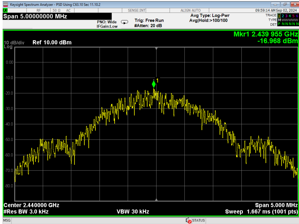
43, PSD, BLE 2MB, Mid
