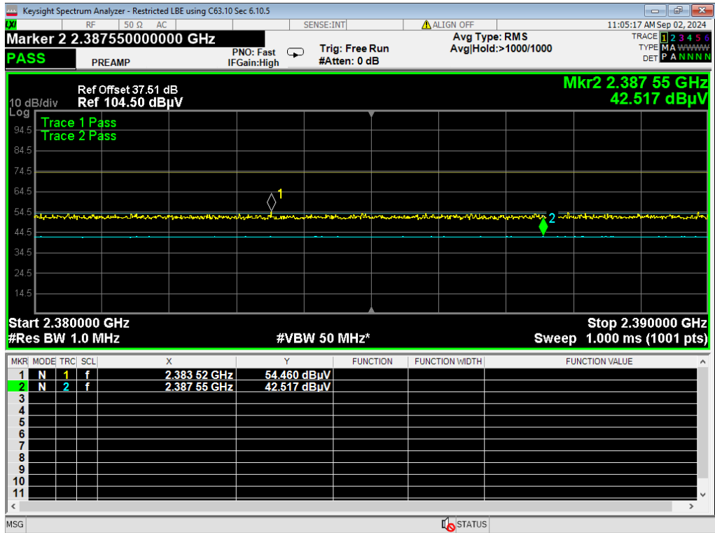
47, LBE Restricted, BLE 2MB
