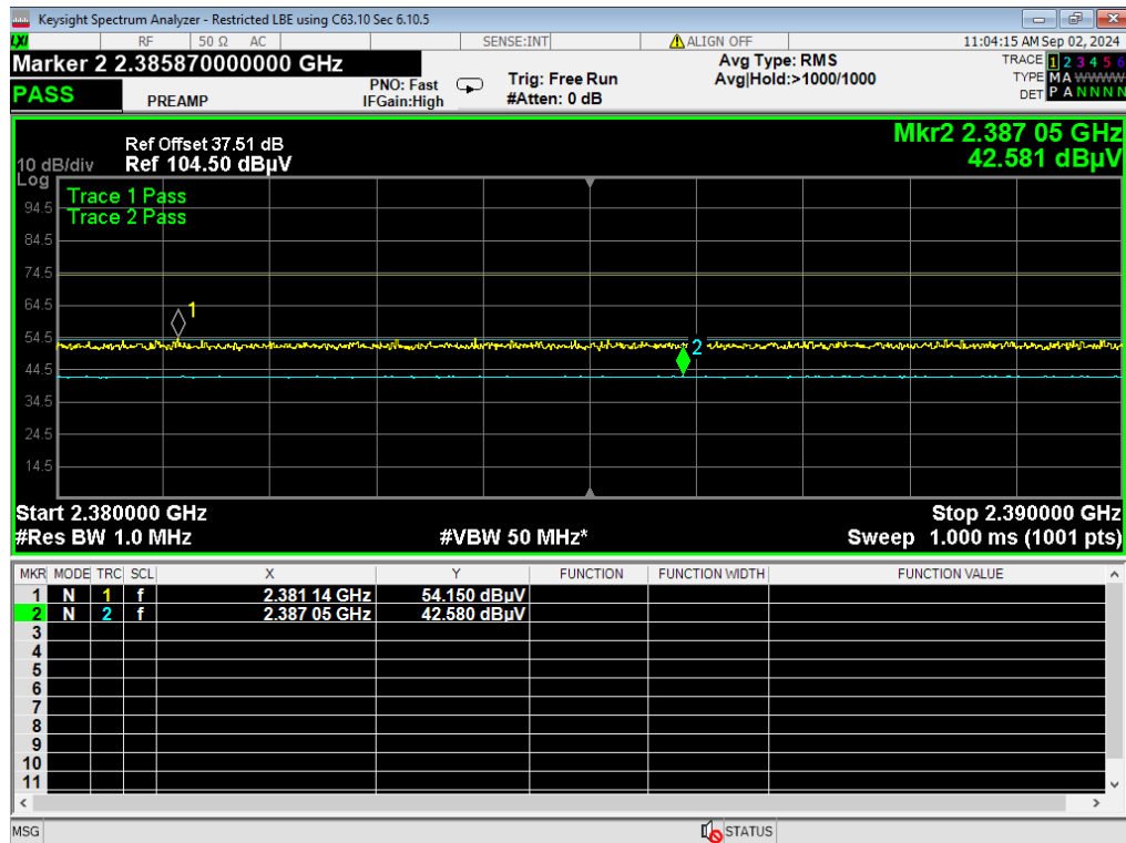
31, LBE Restricted, BLE 1MB
