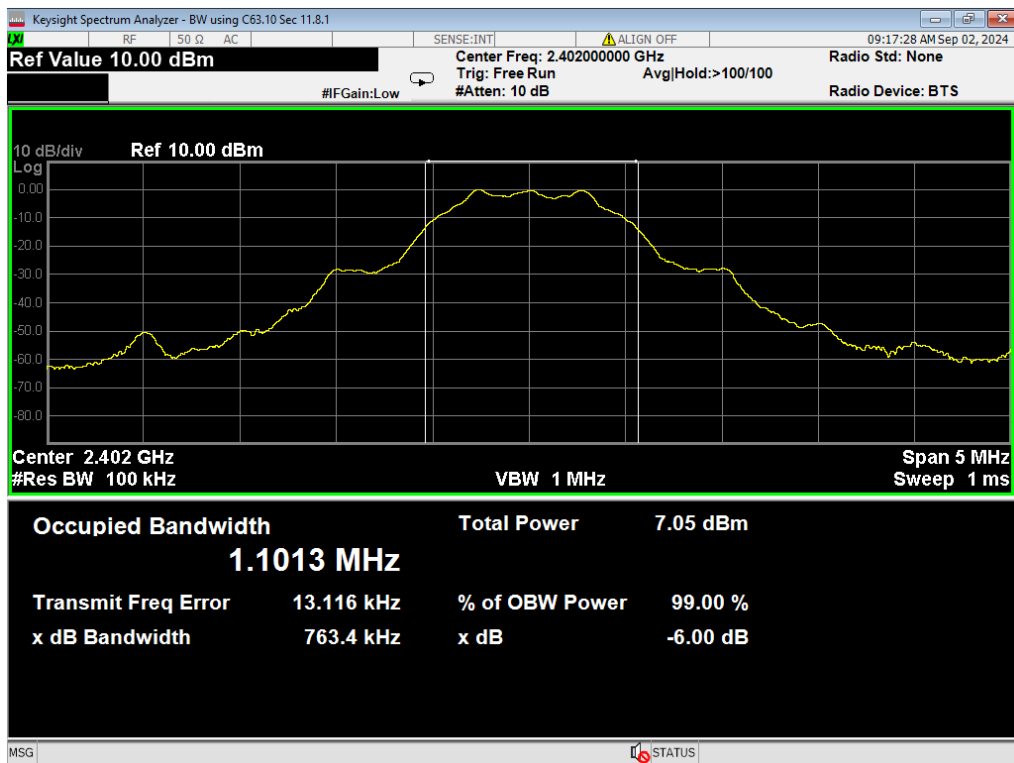
23, 6dB Bandwidth, BLE 1MB, Low
