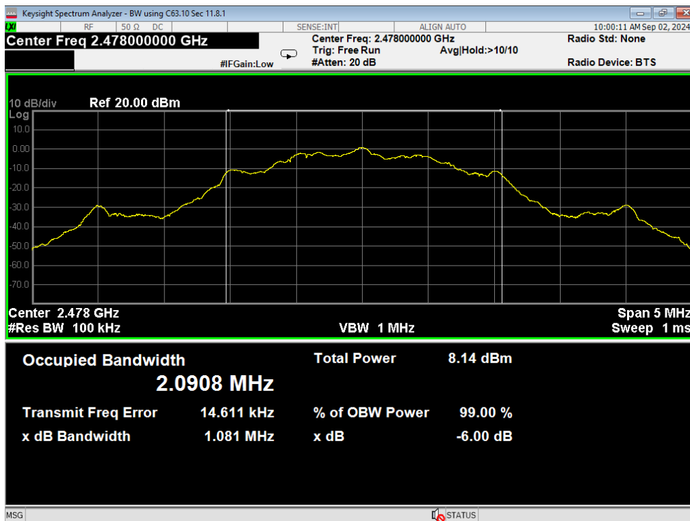
41, 6dB Bandwidth, BLE 2MB, High
