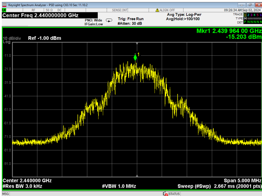
27, PSD, BLE 1MB, Mid
