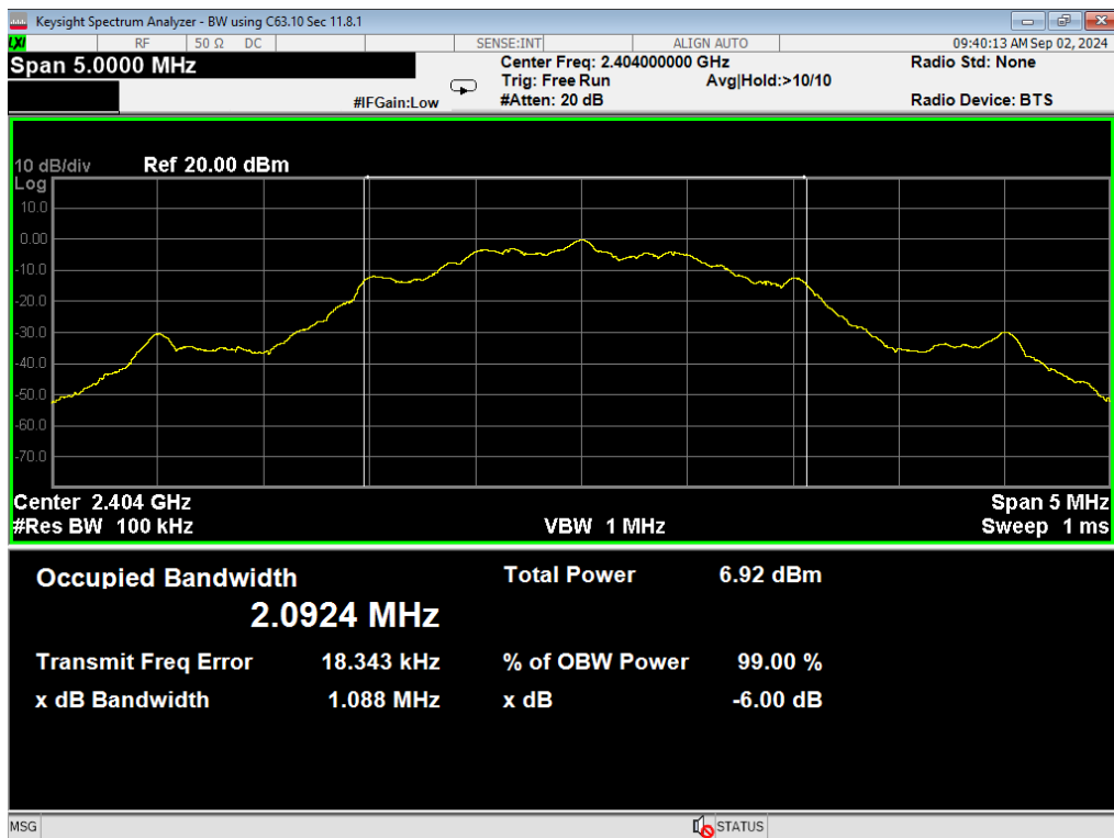
39, 6dB Bandwidth, BLE 2MB, Low
