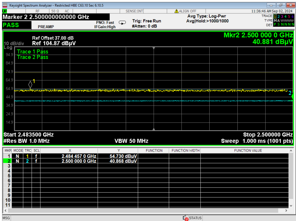
48, HBE Restricted, BLE 2MB
