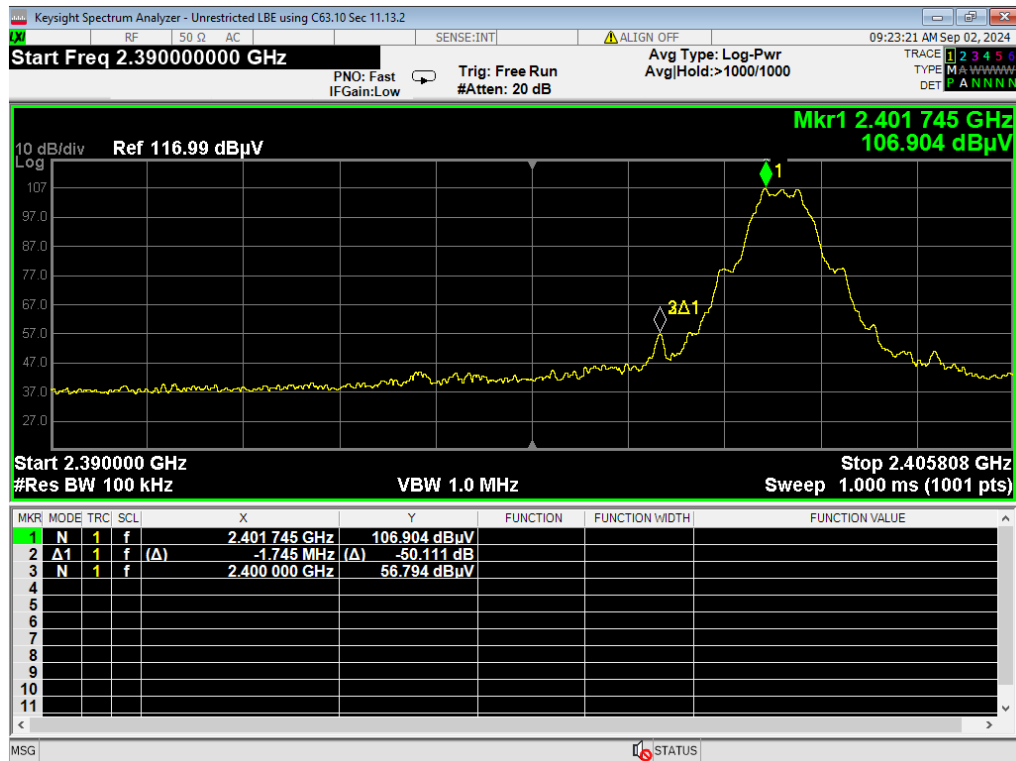
29, LBE Unrestricted, BLE 1MB
