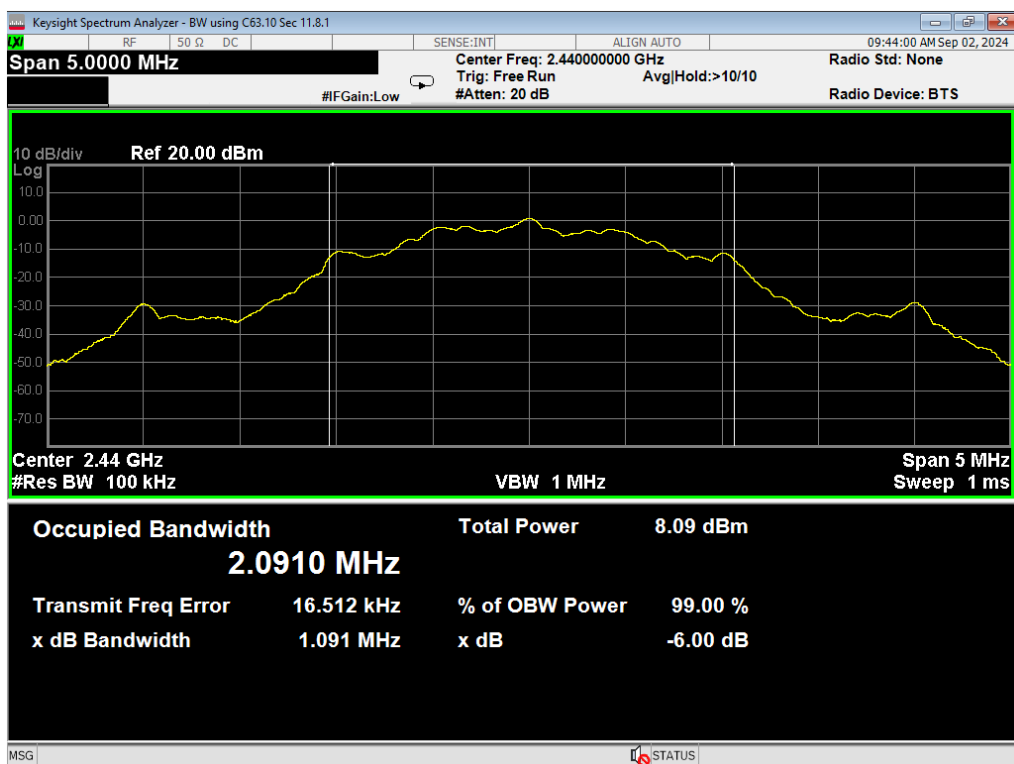
40, 6dB Bandwidth, BLE 2MB, Mid
