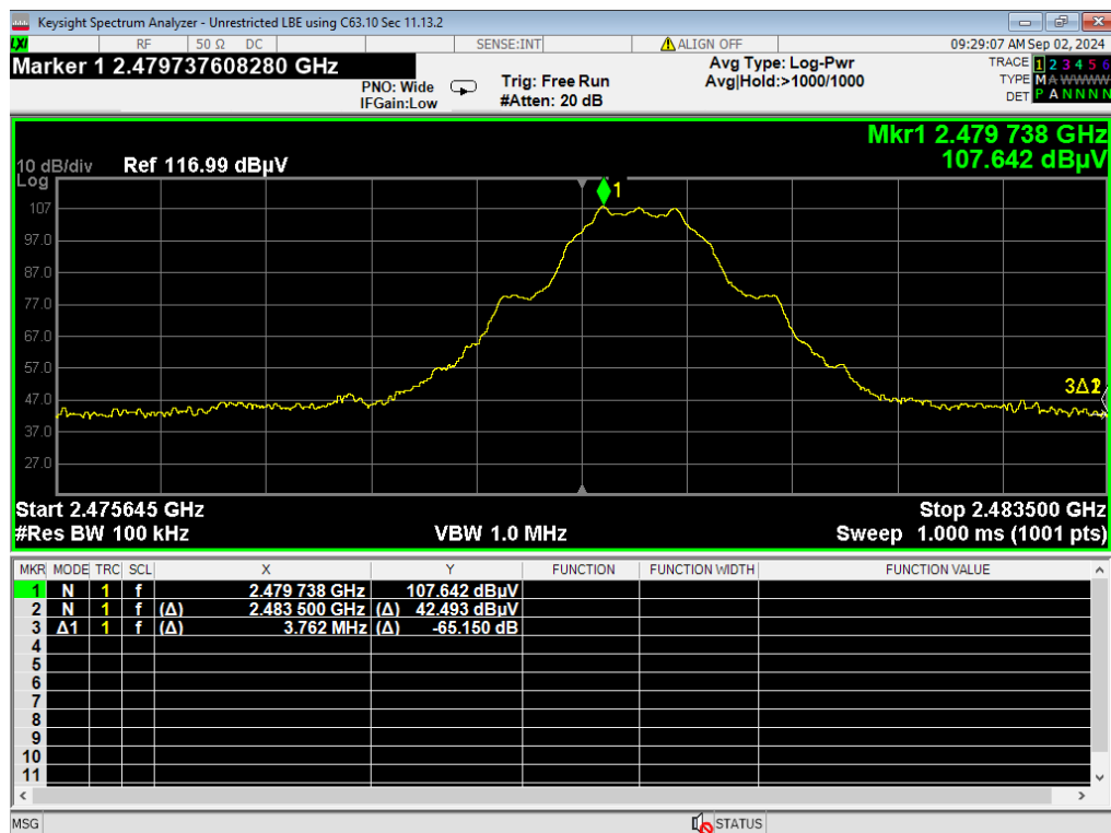
30, HBE Unrestricted, BLE 1MB
