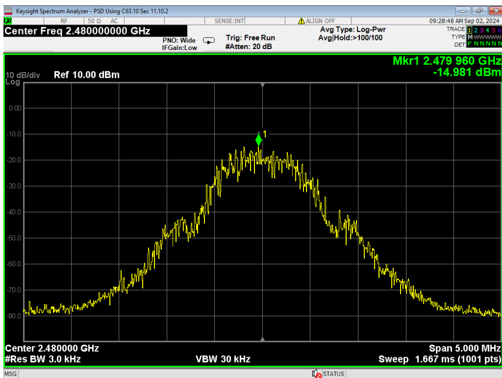
28, PSD, BLE 1MB, High
