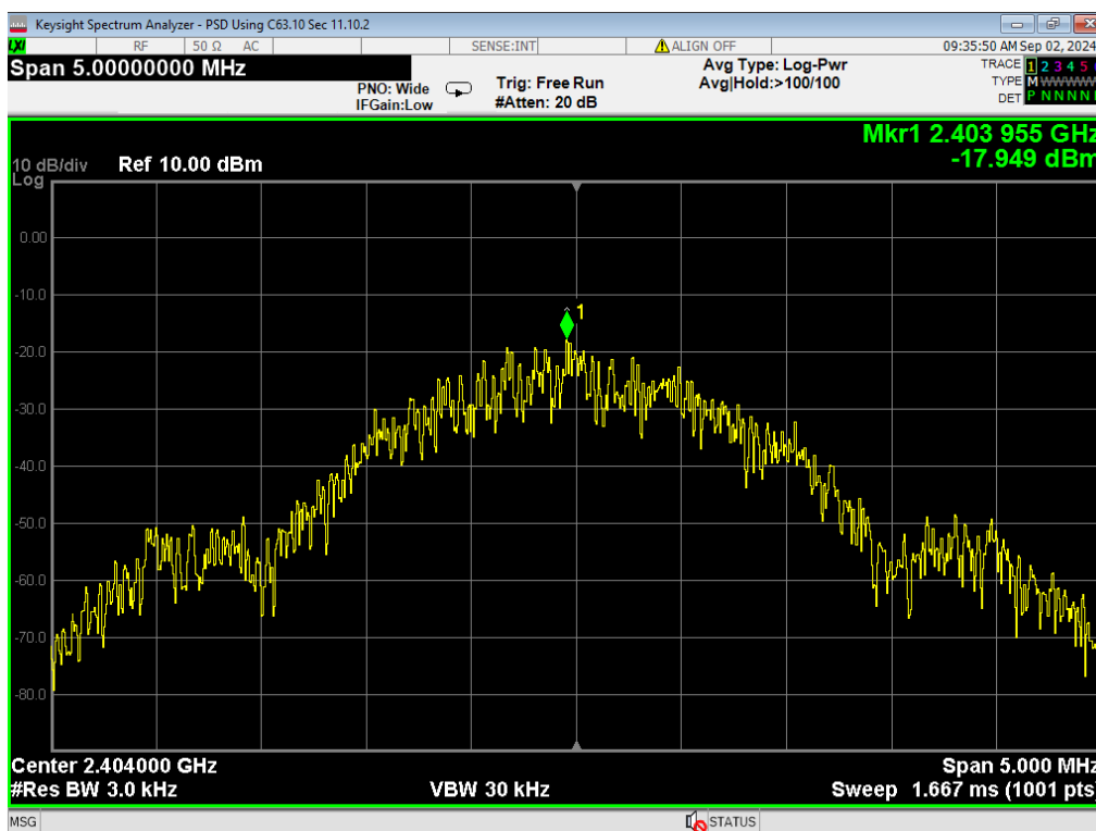
42, PSD, BLE 2MB, Low
