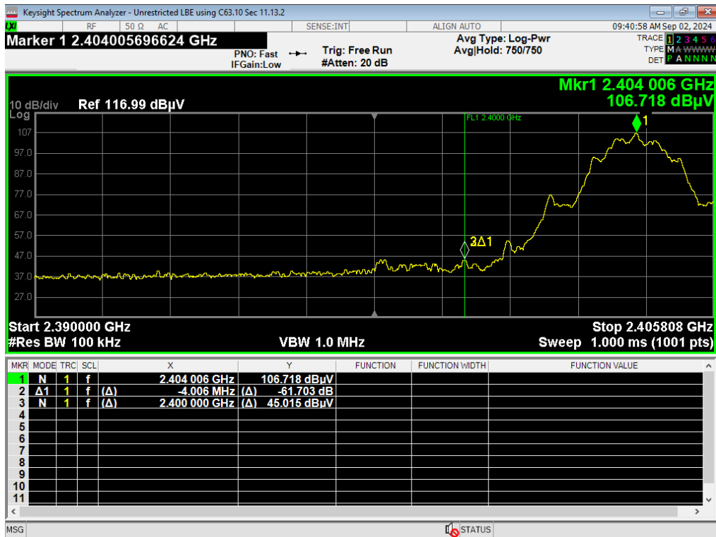
45, LBE Unrestricted, BLE 2MB
