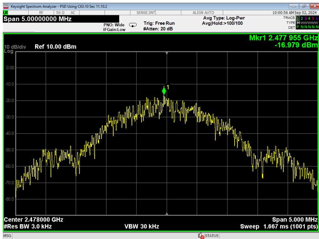
44, PSD, BLE 2MB, High
