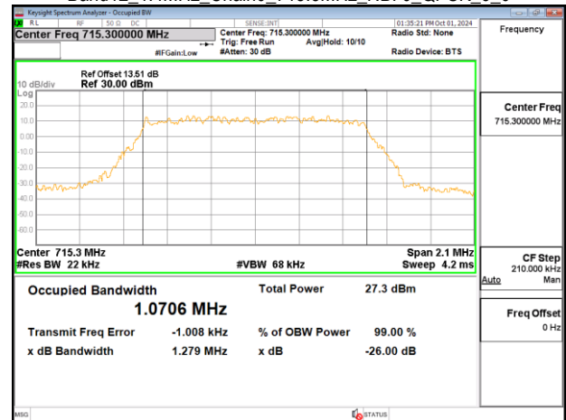
Band12 1.4MHz_Chain0 715.3MHz_NBI 0_QPSK 6_0
