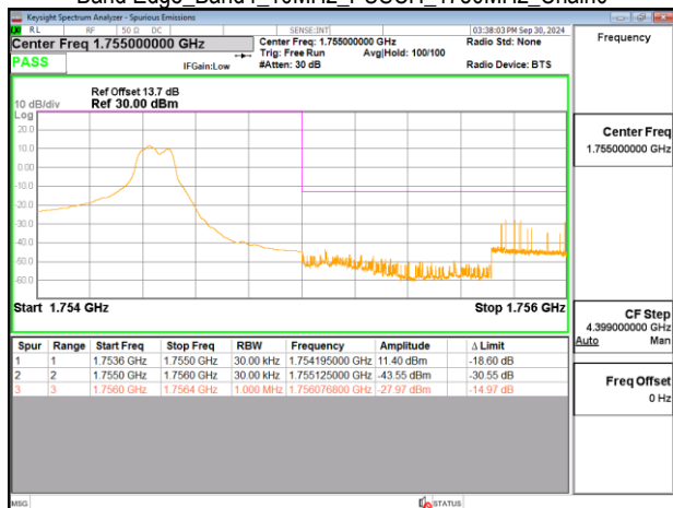
Band Edge_Band4_10MHz_PUSCH_1750MHz_Chain0
