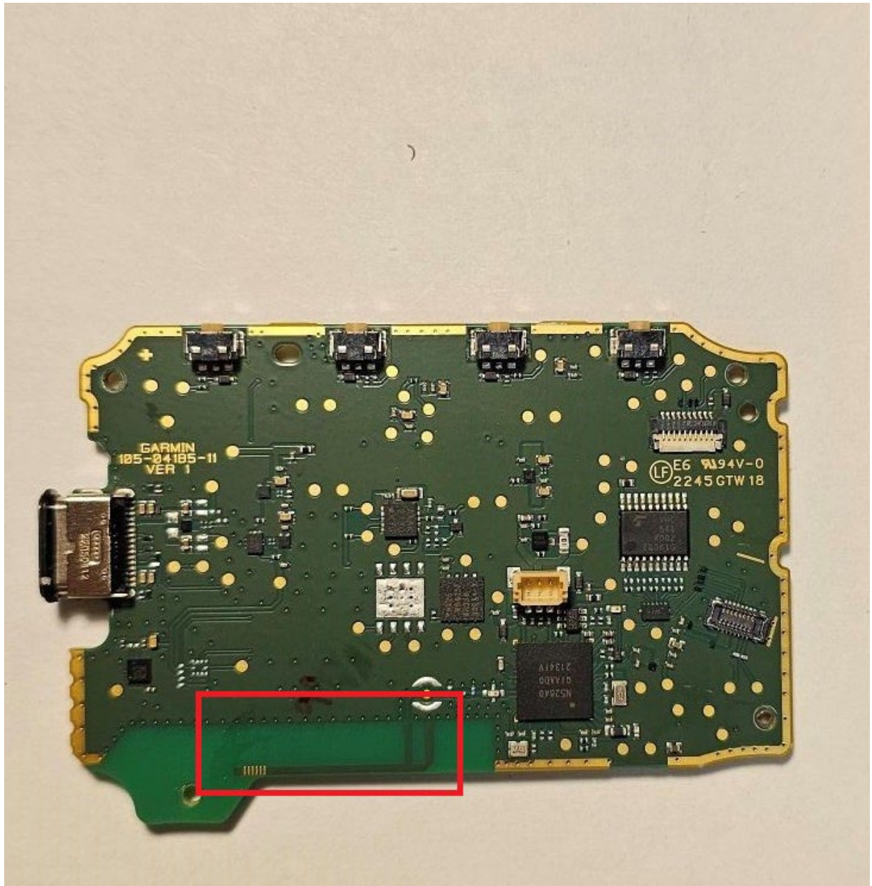
2.4 GHz Antenna
