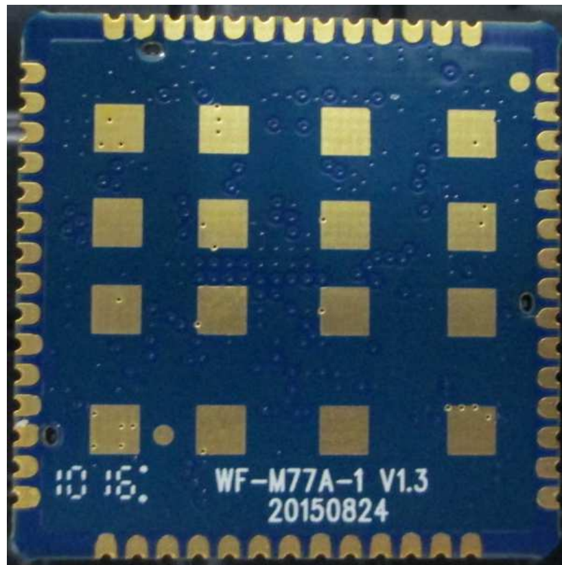
Module (B-side)
