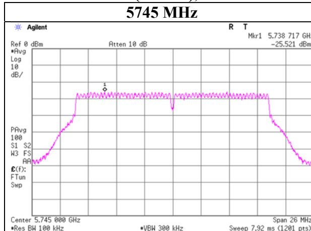
11n-20 (MIMO), Ant 0
