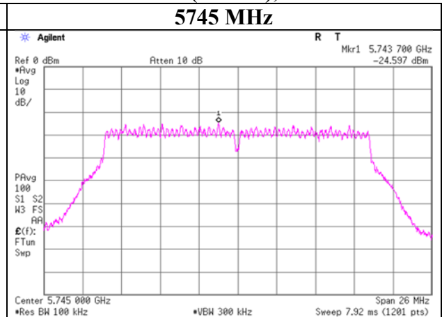
11ac-20 (MIMO), Ant 1
