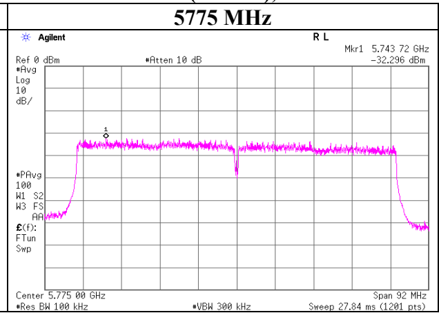
11ac-80 (MIMO), Ant 1
