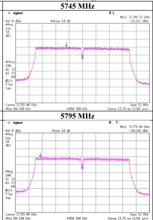
11ac-40 (MIMO), Ant 1
