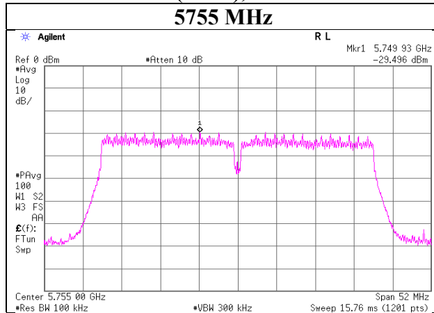
11ac-40 (SISO), Antenna 1
