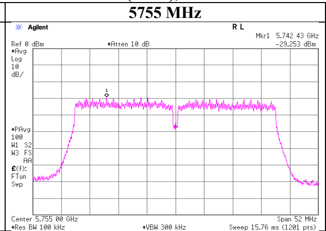
11n-40 (SISO), Antenna 1
