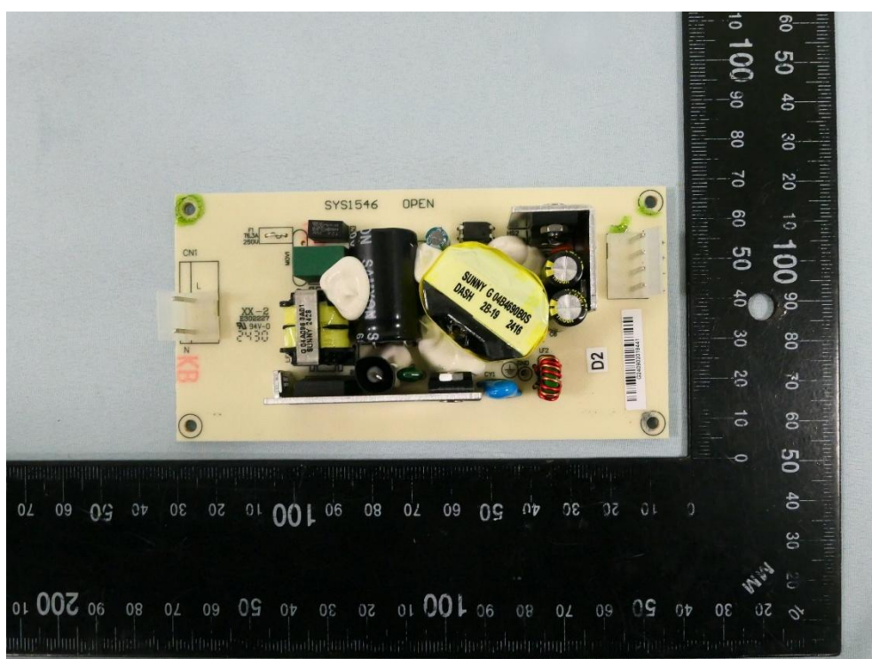
(50) EUT Photo
