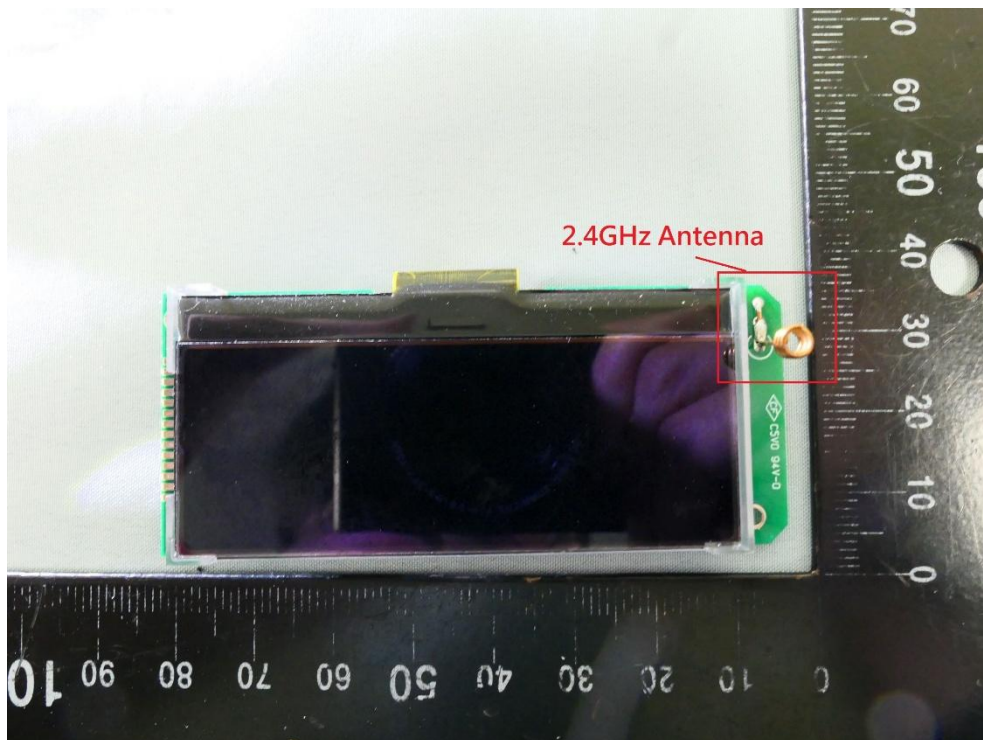
(50) EUT Photo
