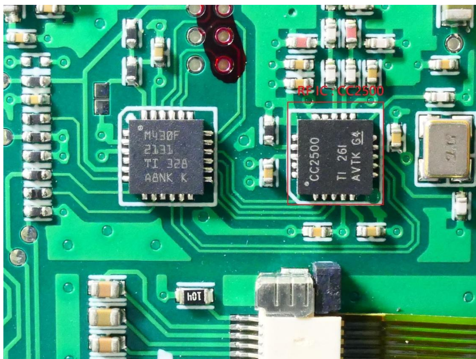
(48) EUT Photo
