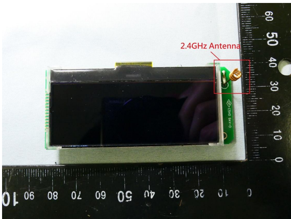
(40) EUT Photo
