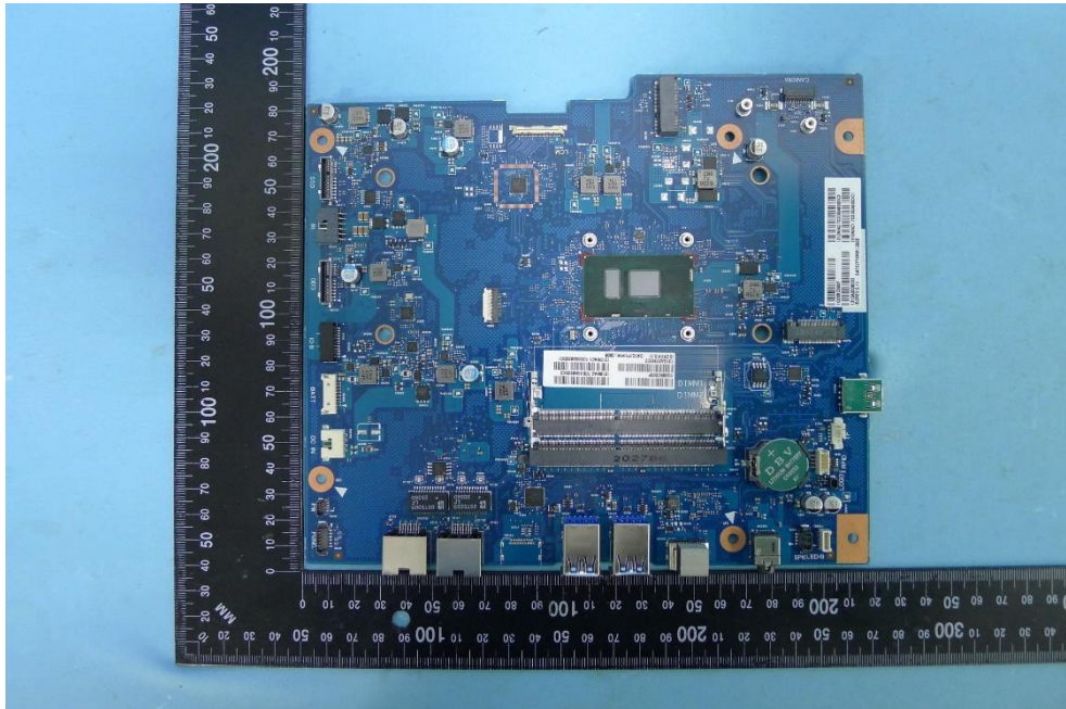
(40) EUT Photo
