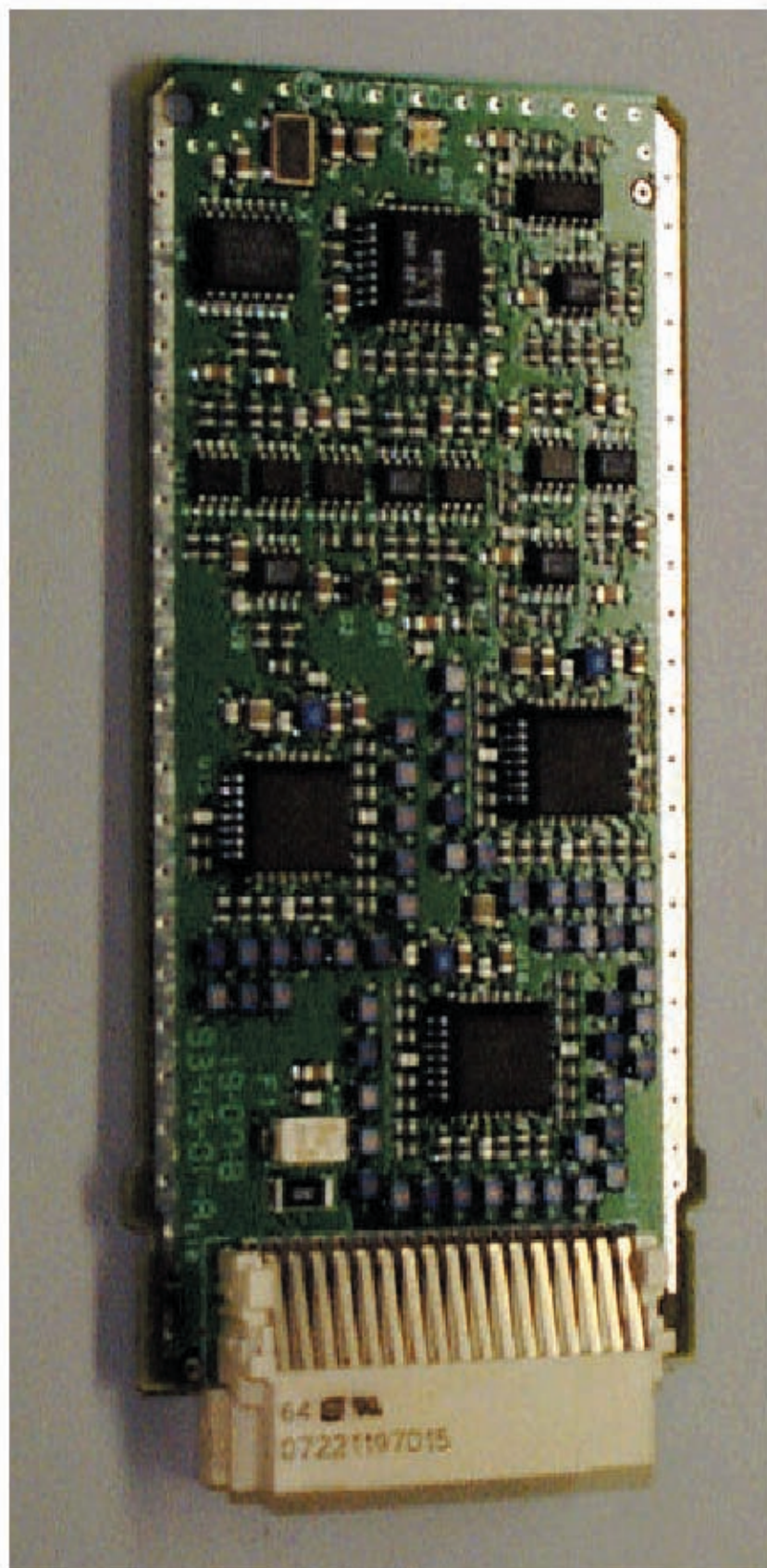
IHET5AP2 SC4812ETL 800MHz CCD Front
