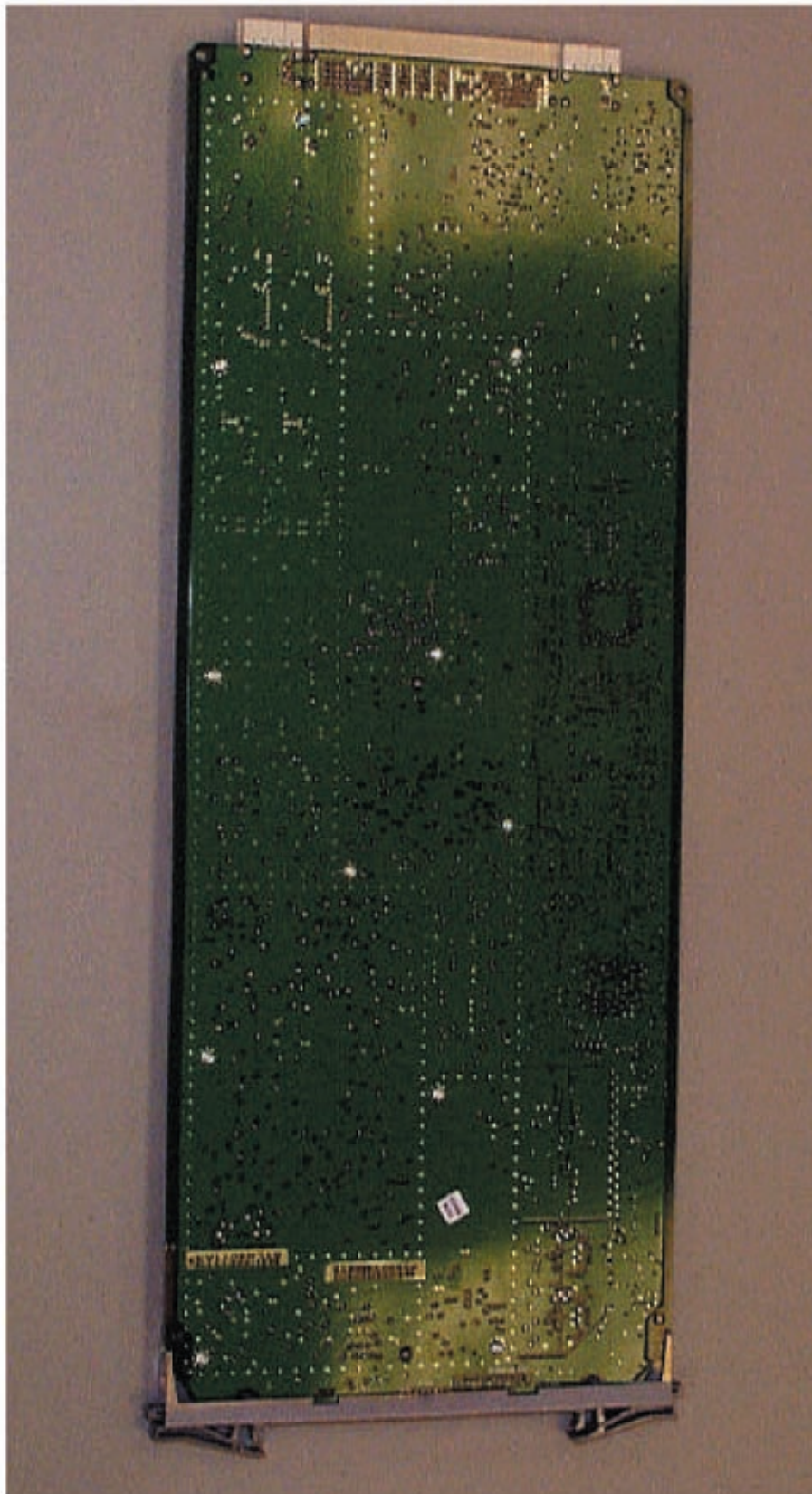
IHET5AP2 SC4812ETL 800 MHz BBX2 Back
