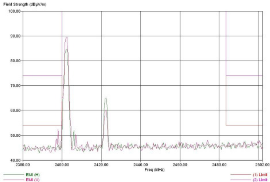
YinTai2 21534 (30 MHz-3 GHz) - Zoom1
