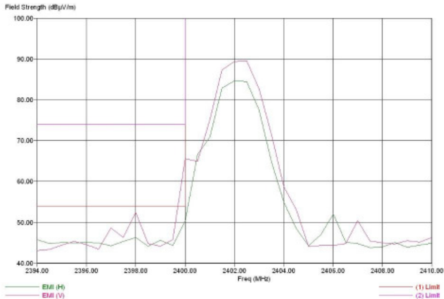
YinTai2 21534 (30 MHz-3 GHz) - Open - Zoom1.1
