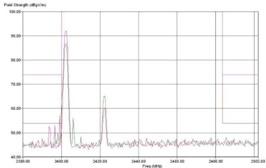
YinTai2 21534 (30 MHz-3 GHz) - Zoom 1
