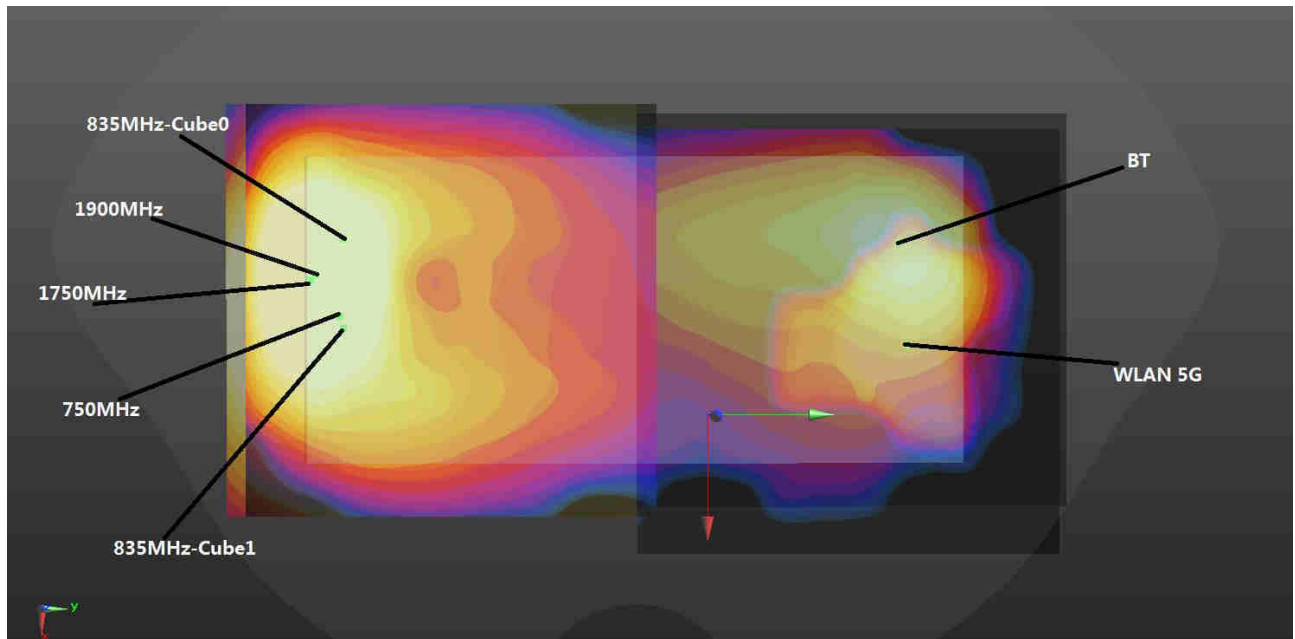
WWAN(5mm)+5GHz(5mm)+BT(5mm)
