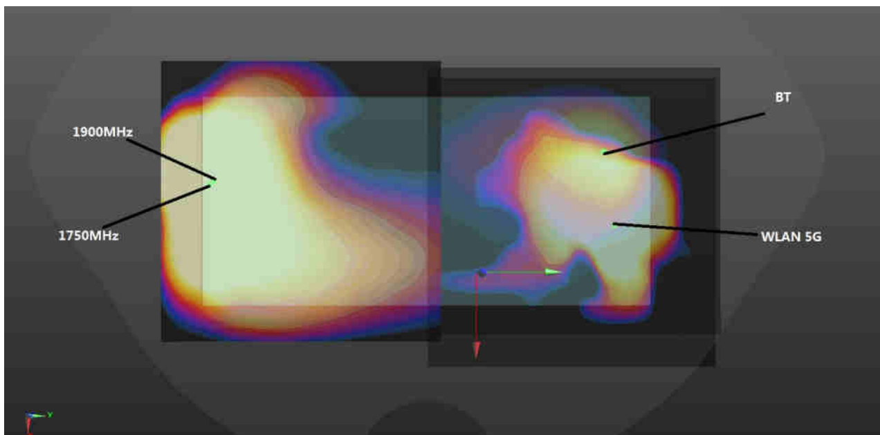
WWAN(23mm)+5GHz(23mm)+BT(23mm)
