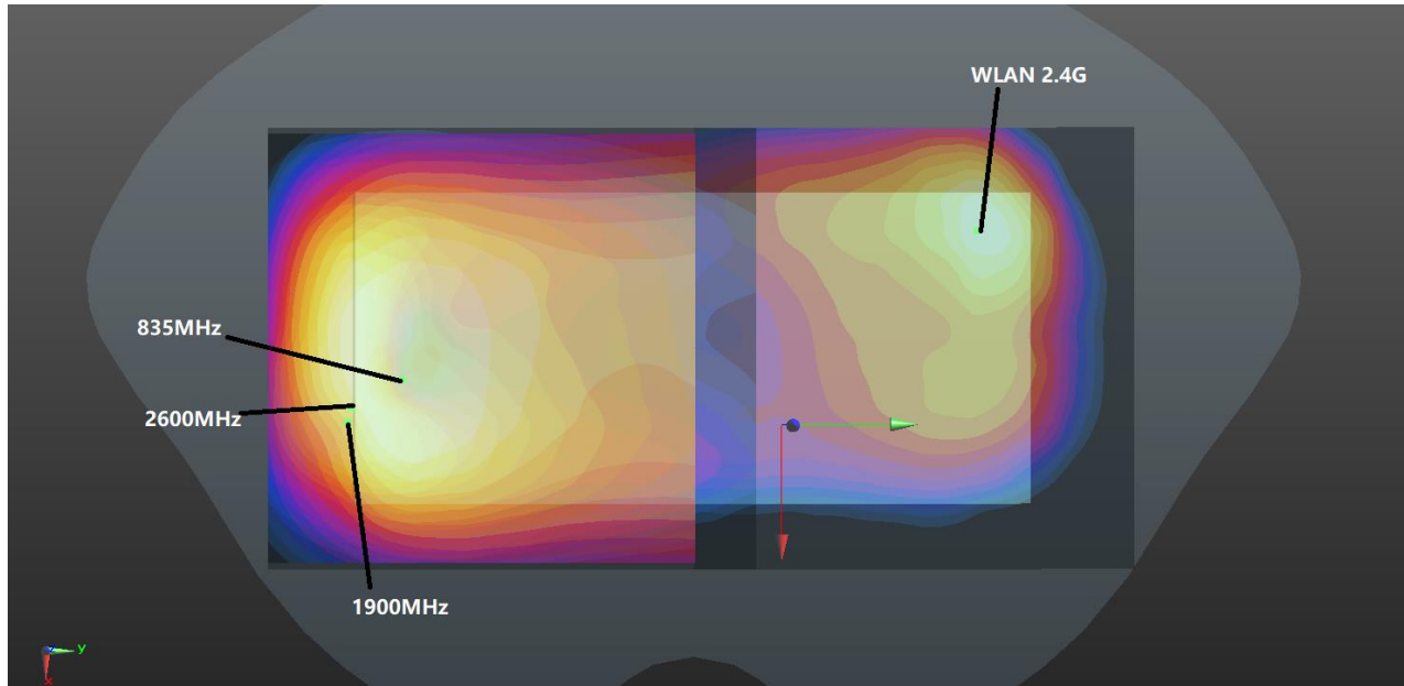
Back(5mm)+WLAN2.4GHz(5mm)
