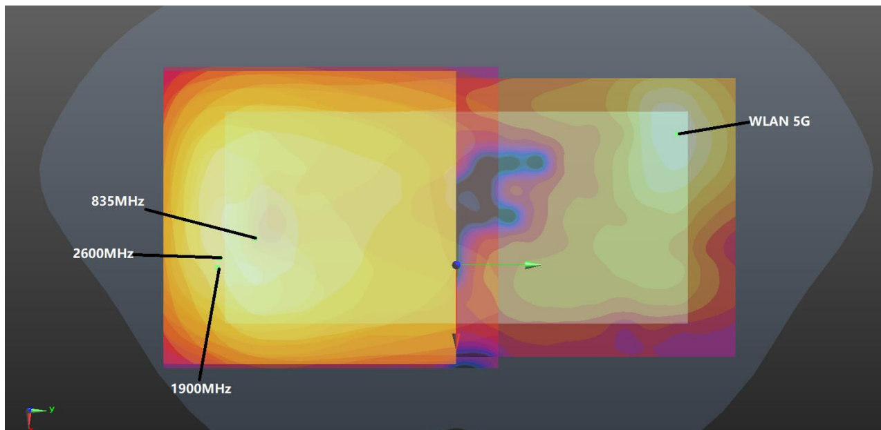
Back(5mm)+ WLAN5GHz(5mm)
