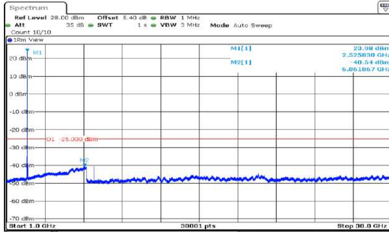
Band7-20MHz-QPSK-21100-1RB#0-Range2:1000~30000MHz
