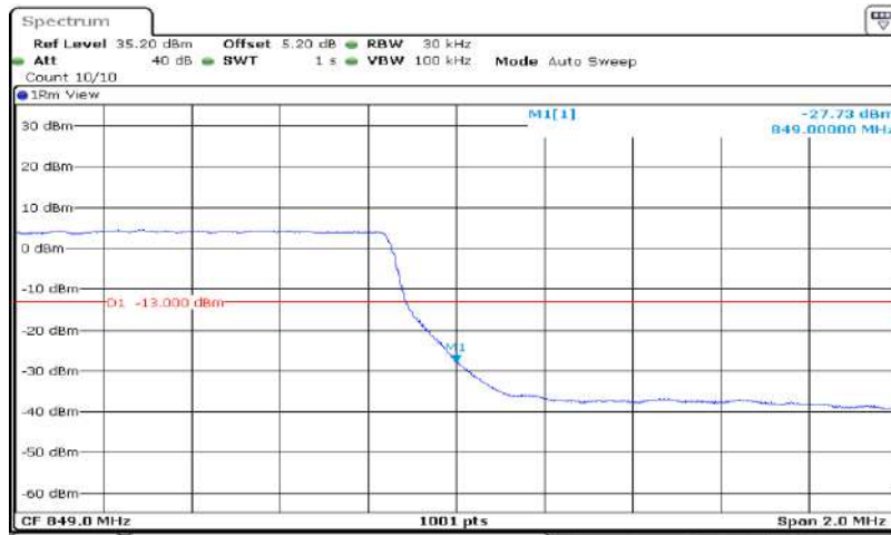
Band5-3MHz-QPSK-20635-15RB#0
