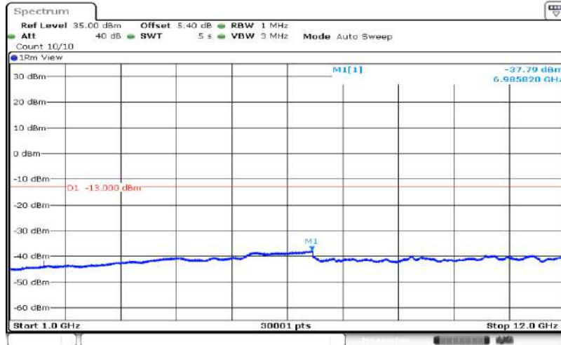
Band5-10MHz-QPSK-20525-1RB#0-Range2:1000~12000MHz
