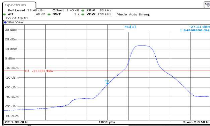
Band2-5MHz-QPSK-18625-25RB#0
