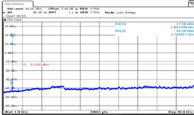
Band2-20MHz-QPSK-19100-1RB#0-Range2:1000~20000MHz
