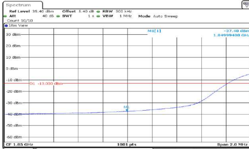
Band2-20MHz-16QAM-18700-100RB#0
