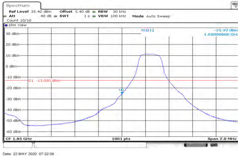
Band2-3MHz-QPSK-18615-15RB#0
