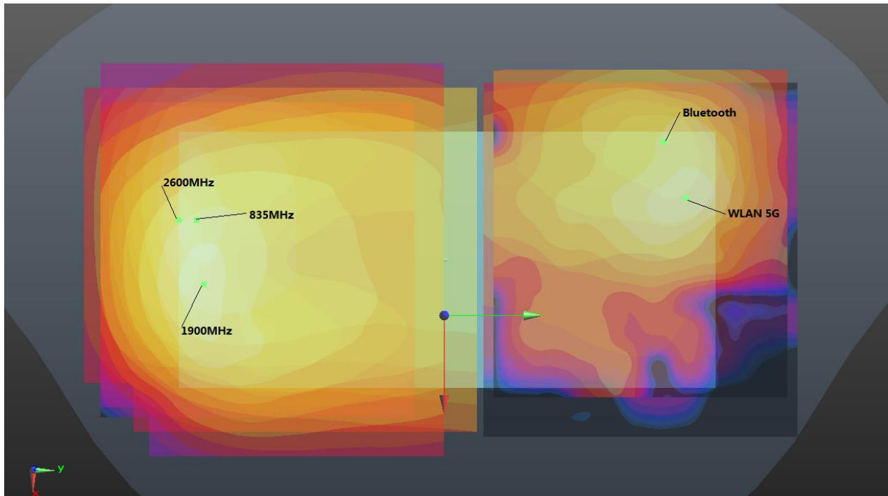
Back(5mm)+BT(5mm)+ WLAN 5G(5mm)
