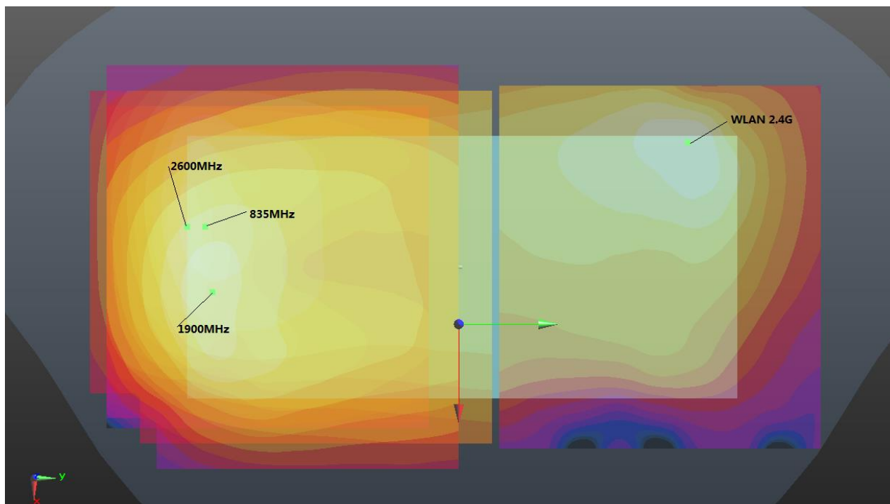
Back(5mm)+WLAN 2.4G(5mm)
