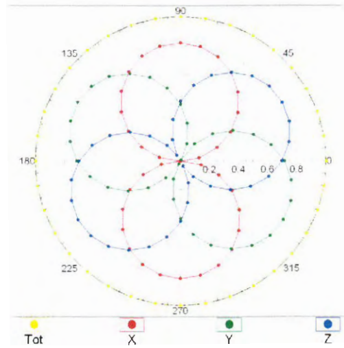
f=1800 MHz,R22
