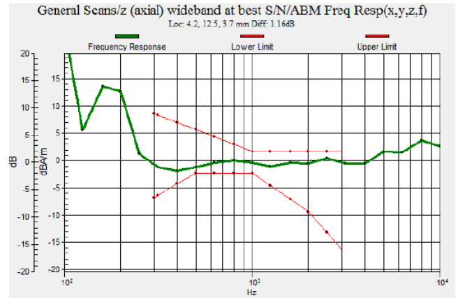
Fig 7.8 CDMA2000 BC10 Ch580
