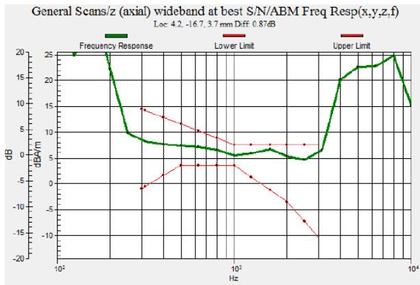
Fig 7.1 GSM850 Ch189
