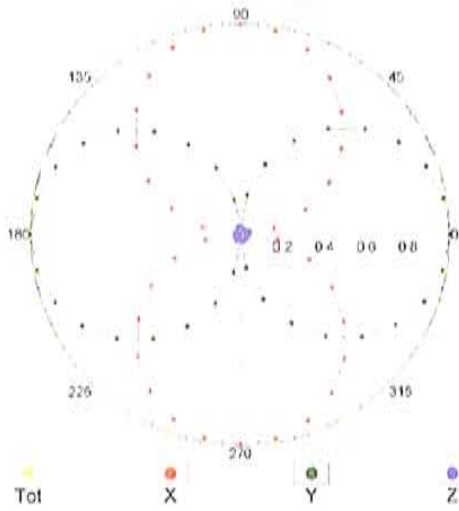
f=600 MHz, TEM, 0^\circ
