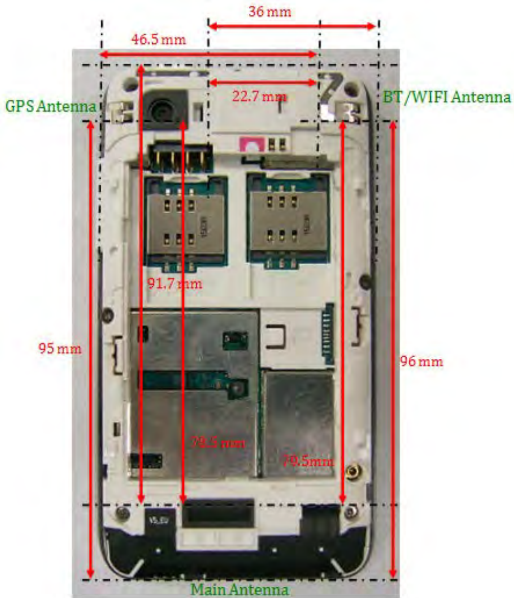
Fig.19 Antenna
