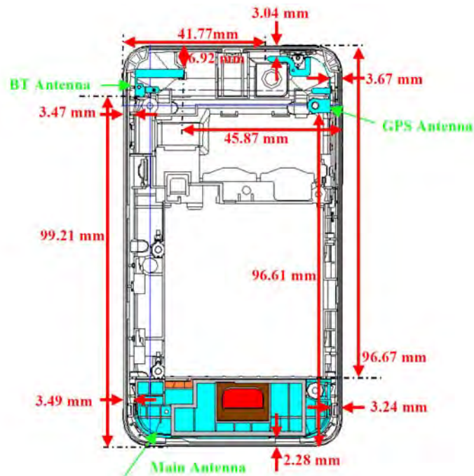
Fig.19 Antenna
