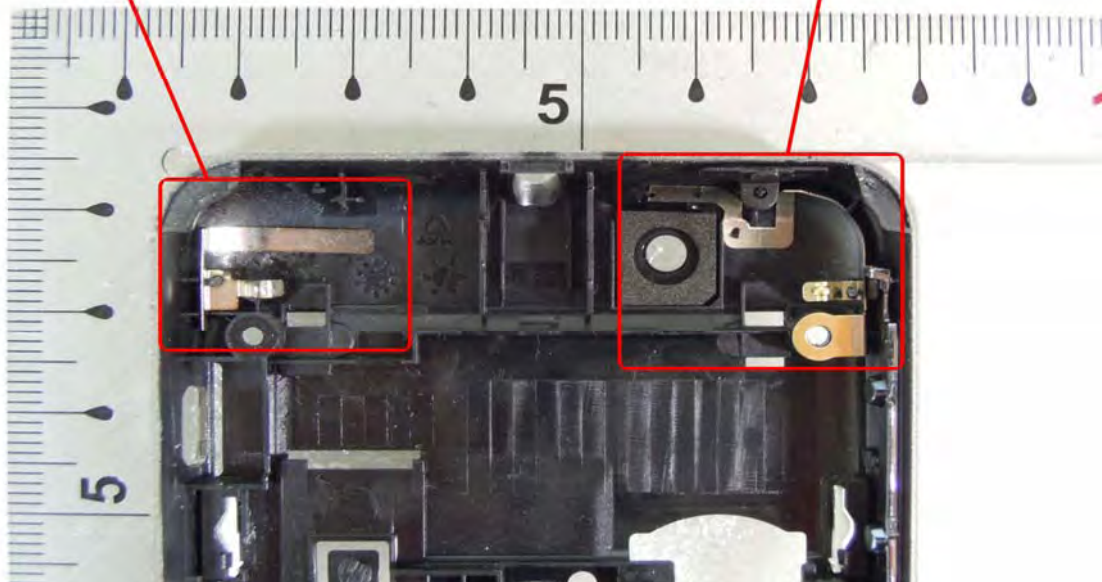
WWAN Antenna
