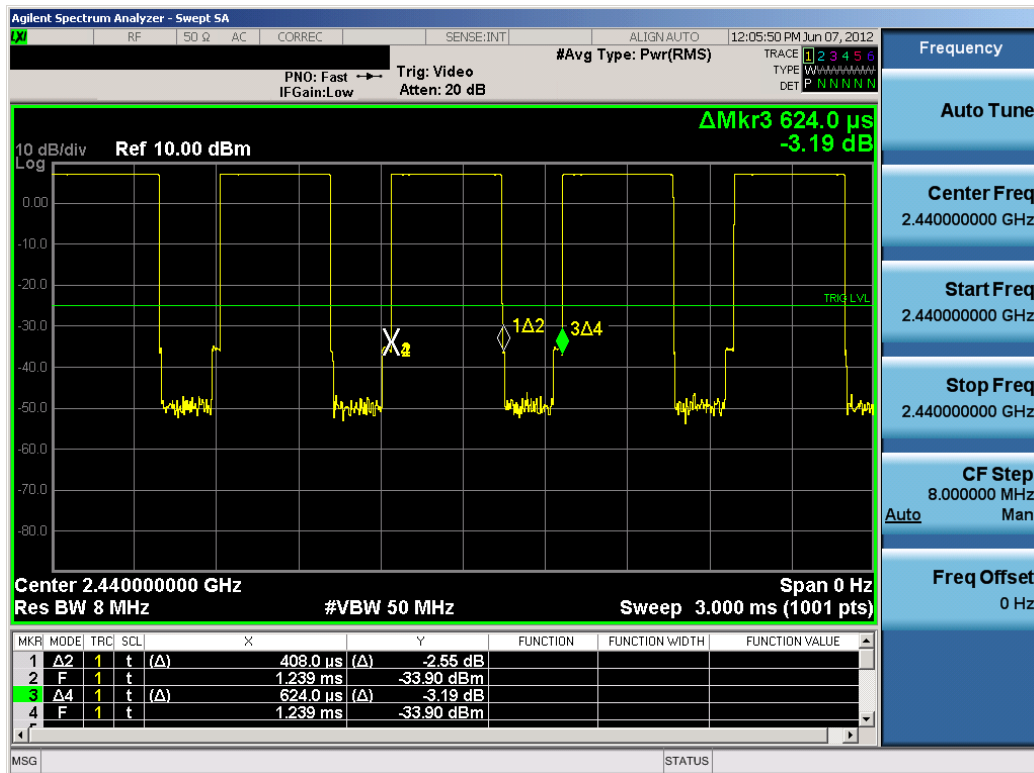
Plot 6-7. Bluetooth LE Pulse Width
