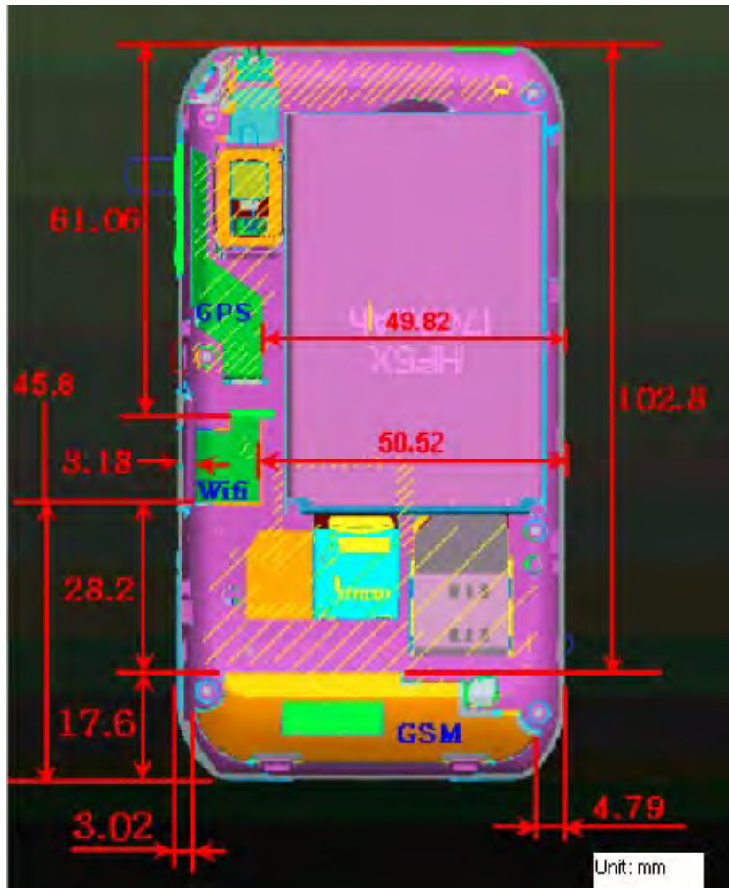
Fig.18 Antenna
