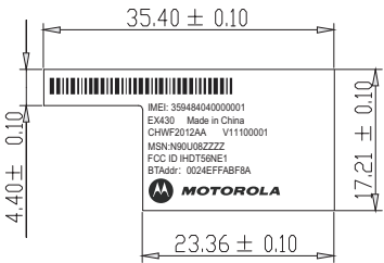
重點尺寸-1
