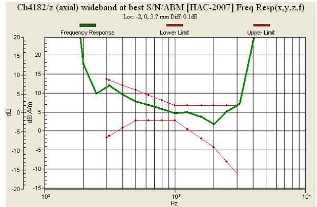
Fig. 9.2 WCDMA Band V Ch4182
