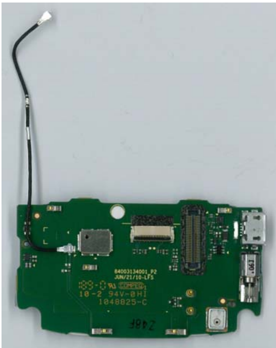
Keypad PCB Bottom
