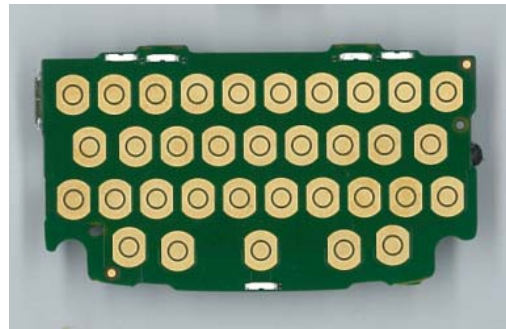
Keypad PCB TOP
