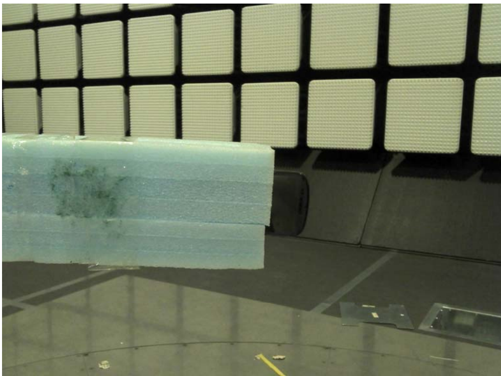
BT & WLAN Y Position
