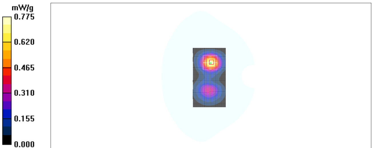
Fig. 34 1900 MHz CH810
