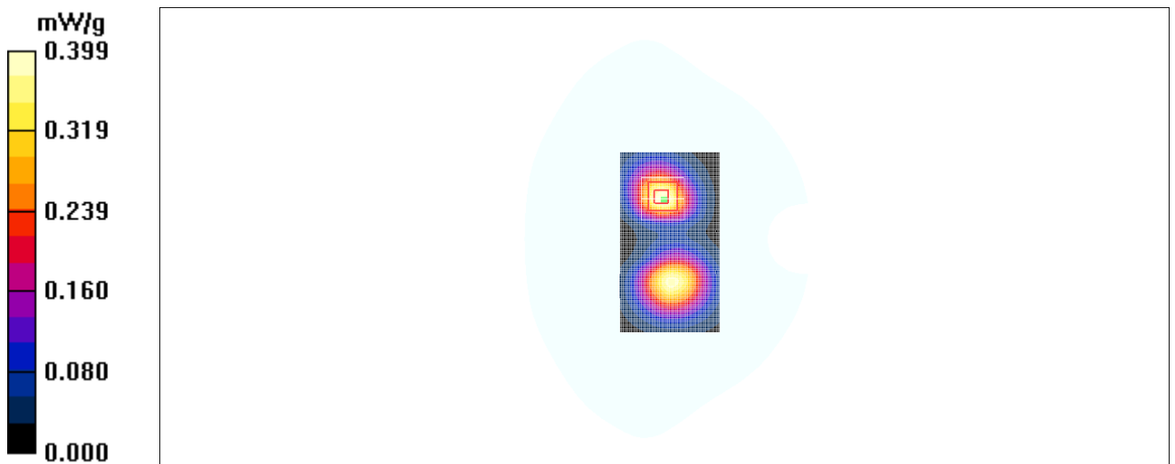
Fig. 37 1900 MHz CH810
