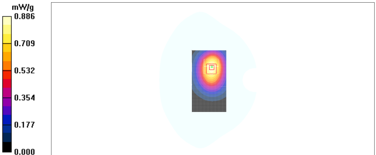
Fig. 33 850 MHz CH251
