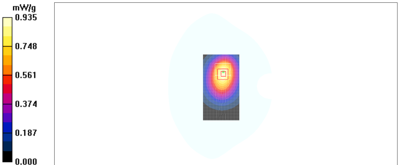
Fig. 42 850 MHz CH251
