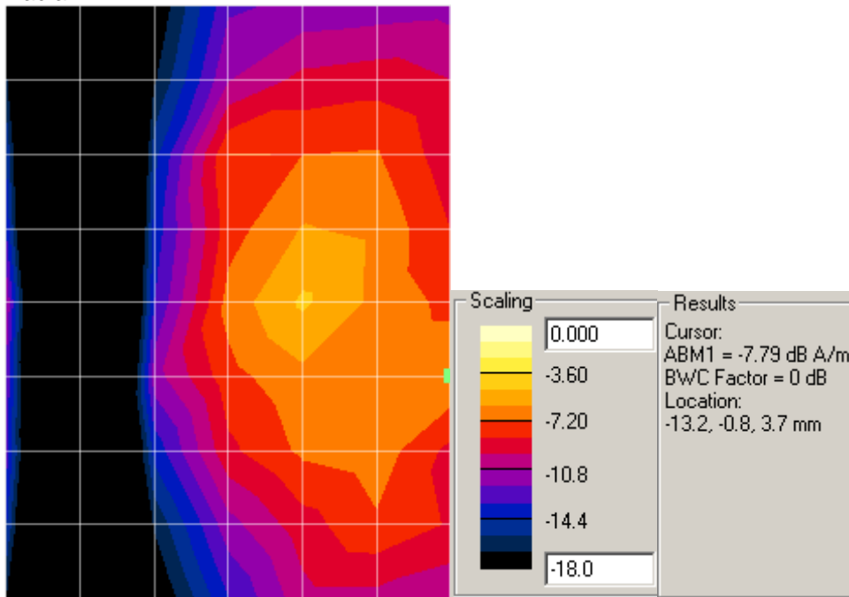
Radial1 – ABM1
